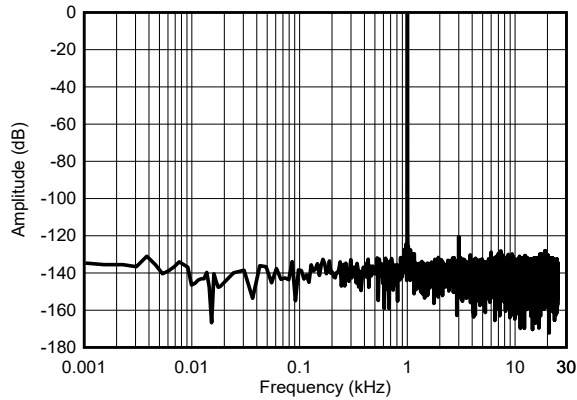
图 6-18. Full-Scale Input FFT
