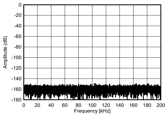
图 6-8. Shorted Input FFT
