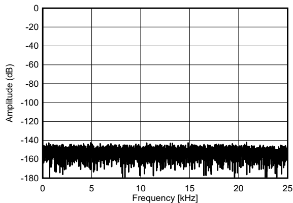
图 6-6. Shorted Input FFT
