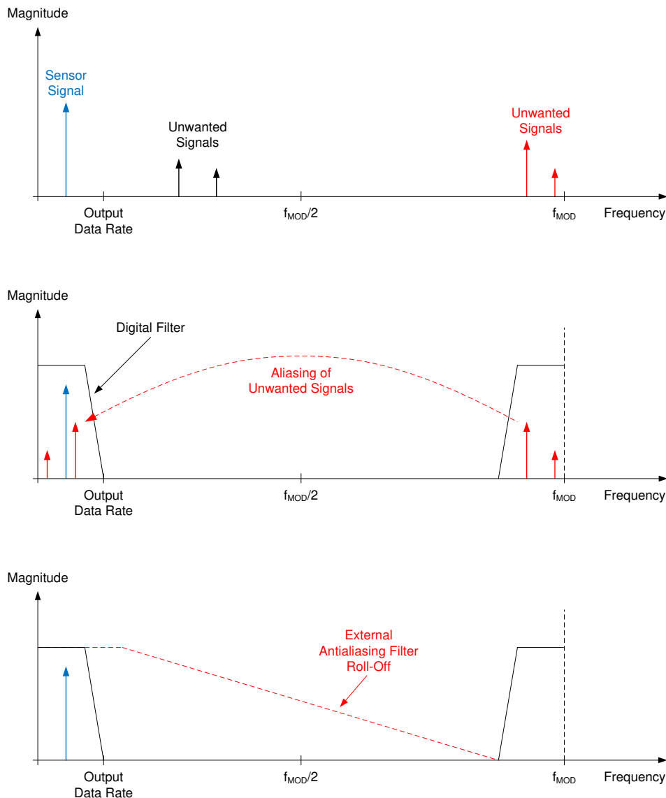
图 95. Effect of Aliasing
