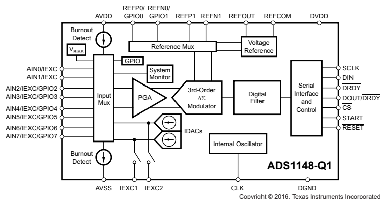
功能方框图
