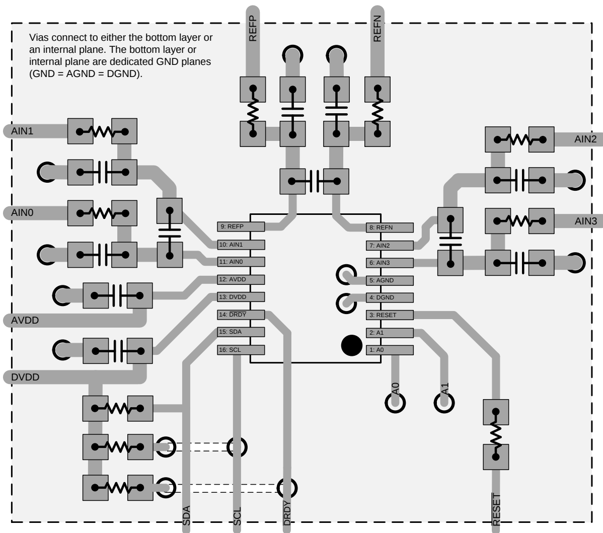
图 48. Layout Example
