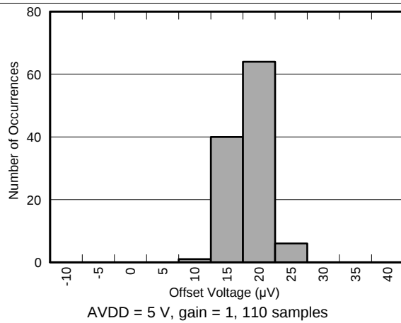
图 8. Offset Voltage Histogram
