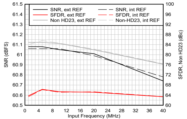
图 5-10. 交流性能与输入频率间的关系
