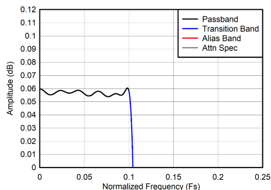
图 6-15. 4 倍抽取率通带纹波响应
