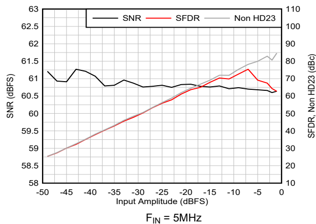
图 5-54. 交流性能与输入幅度间的关系
