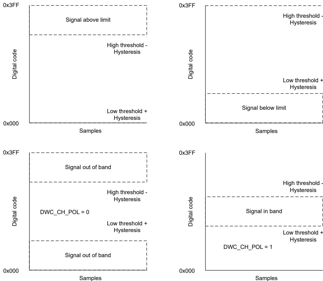
图 6-26. 数字比较器事件监测
