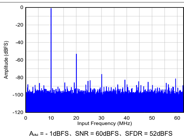
图 7-3. 10MHz FFT (THS4541 FDA)
