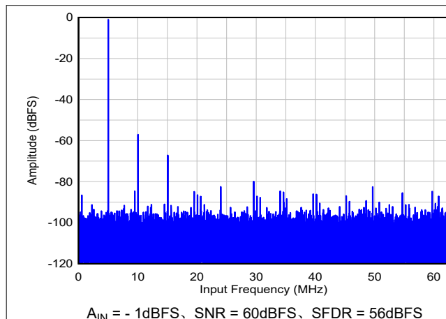
图 7-2. 5MHz FFT (THS4541 FDA)
