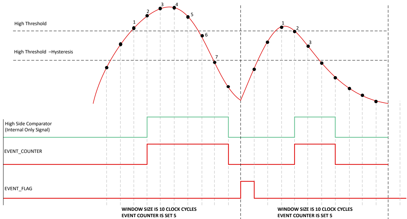
图 6-28. 窗口监测
