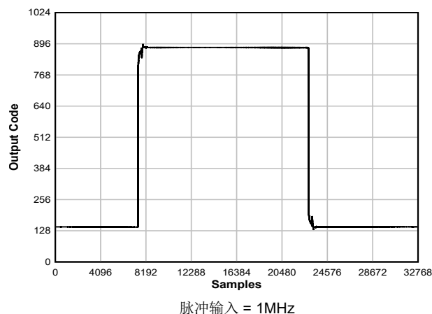
图 5-39. 脉冲响应
