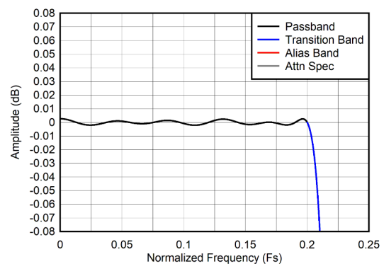
图 6-13. 2 倍抽取率通带纹波响应
