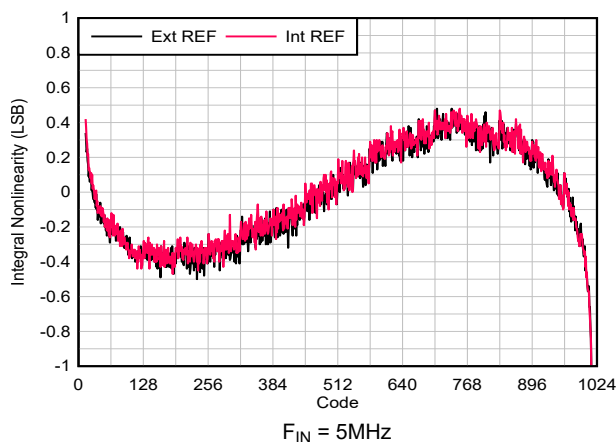
图 5-16. INL 与 ADC 代码间的关系
