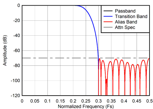
图 6-12. 2 倍抽取率频率响应
