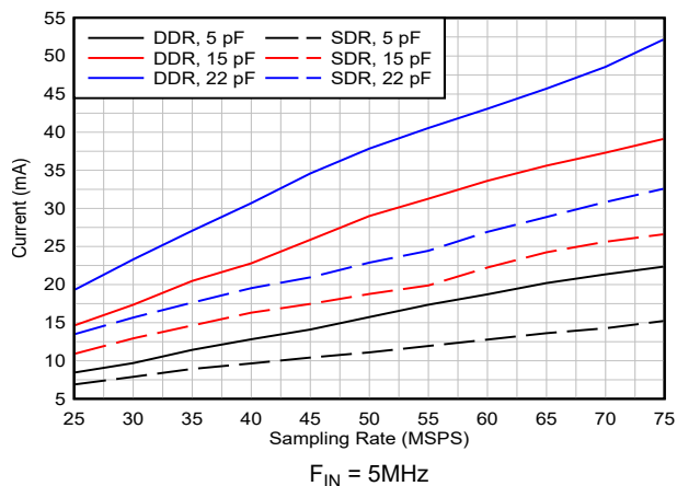
图 5-43. I_{IOVDD} 电流与负载电容间的关系
