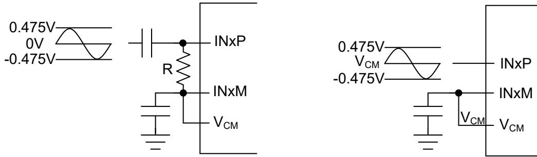
图 7-3. 单端模拟输入：交流耦合 ( 左 ) 和直流耦合 ( 右 )
