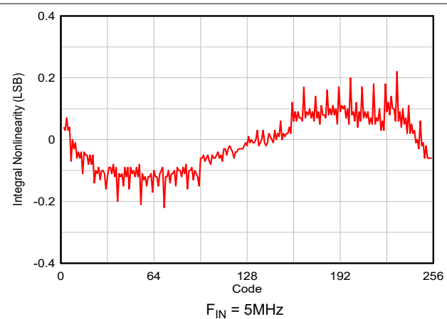
图 6-30. INL 与 ADC 代码间的关系
