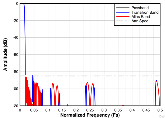
图 7-29. 32 倍抽取率滤波器频率响应
