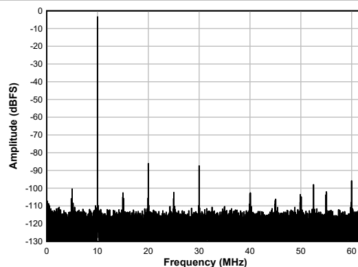
图 5-2. F_{IN} = 10\text{MHz} 时的单音频谱
