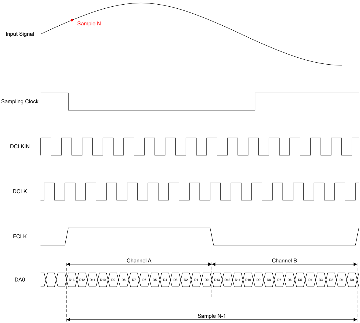
图 6-3. 时序图：1/2 线
