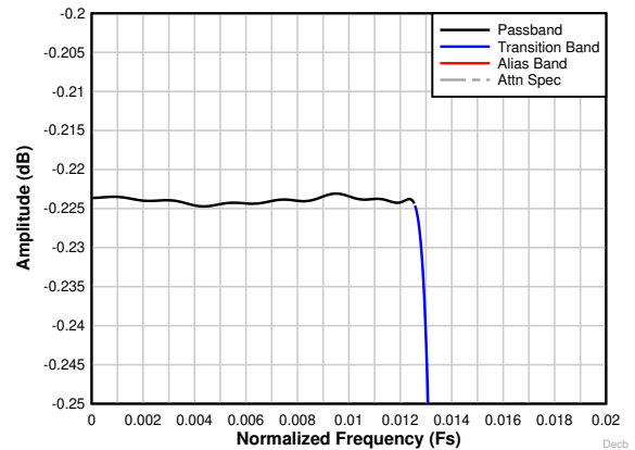
图 7-30. 32 倍抽取率滤波器通带纹波响应
