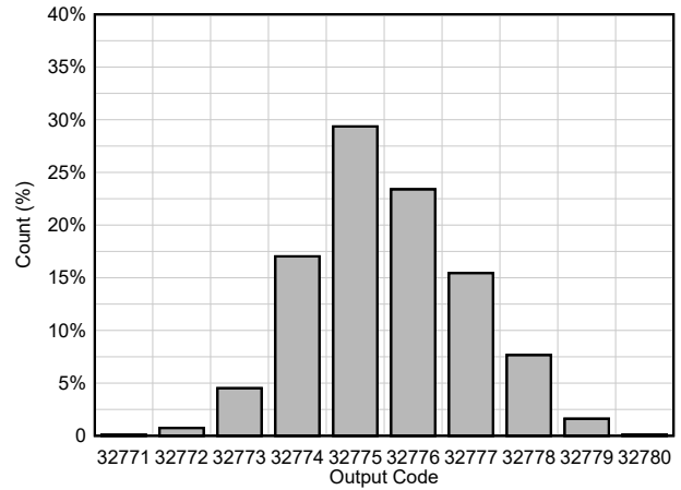
图 6-14. DC Offset Histogram
