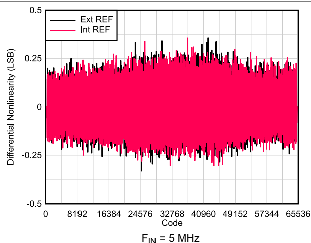
图 6-60. DNL vs Code
