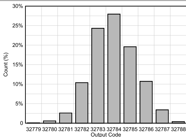
图 6-61. DC Offset Histogram
