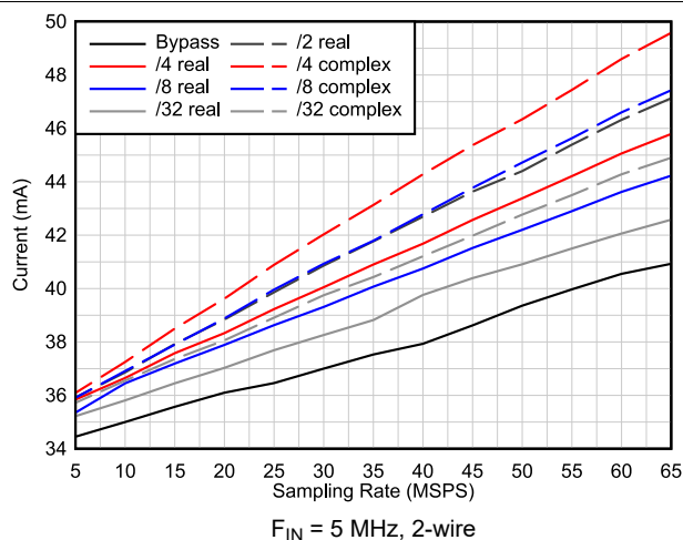
图 6-63. Current vs Decimation
