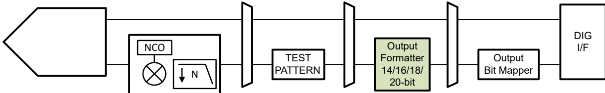
图 8-37. Interface output bit mapper
