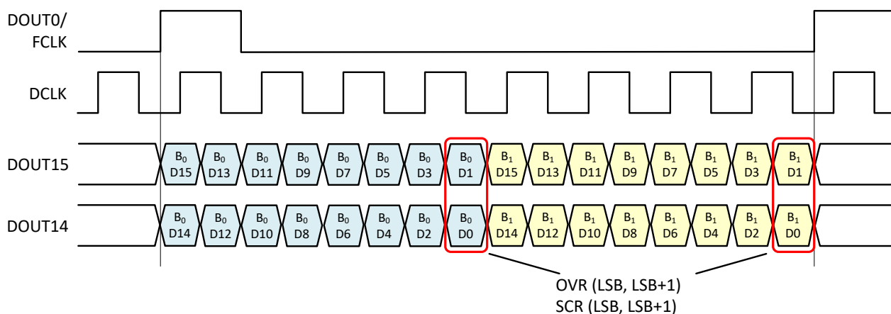
图 8-62. 输出数据替代：<16 条 SLVDS 信道
