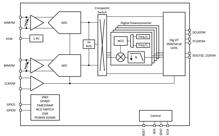
方框图
