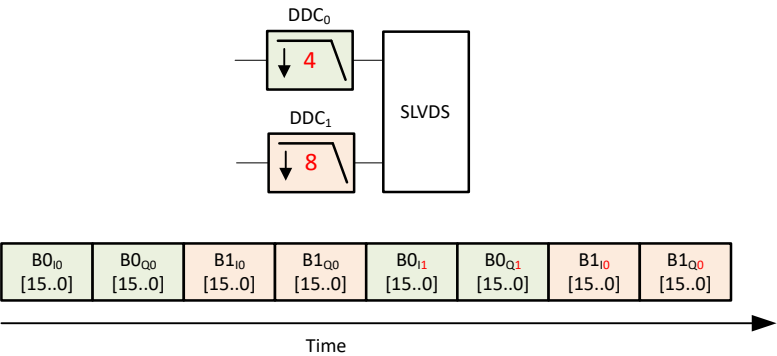
图 8-21. 不等的抽取因子
