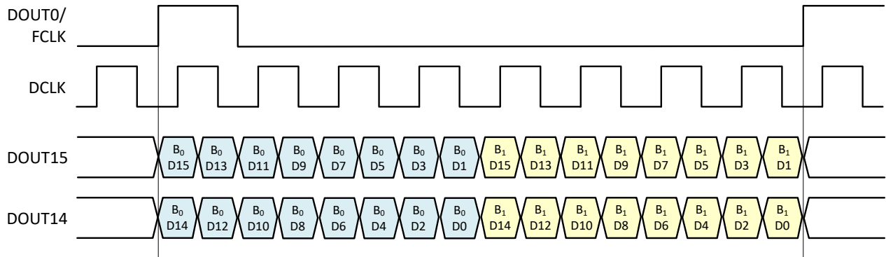
图 8-56. 示例 1 的 SLVDS 帧组装
