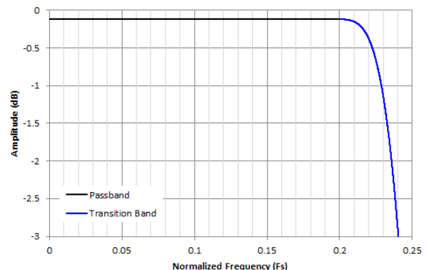
图 8-24. /2 抽取通带纹波响应
