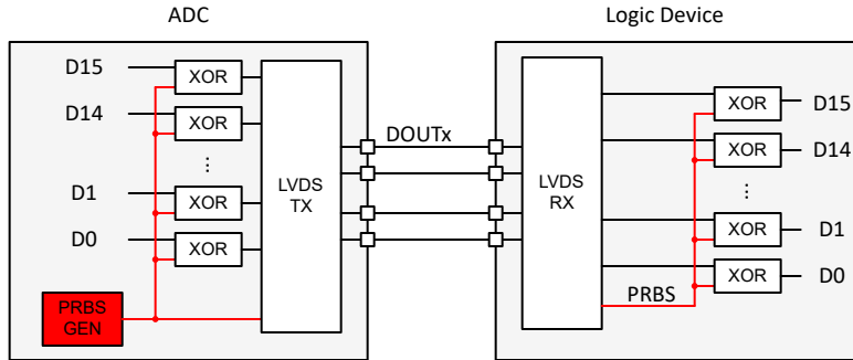
图 8-63. 输出扰频器
