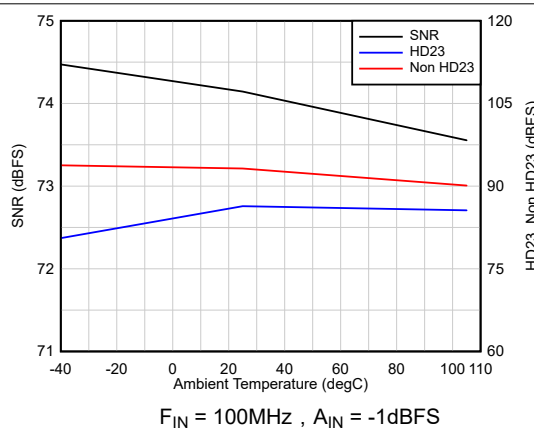
图 6-22. 交流性能与温度间的关系
