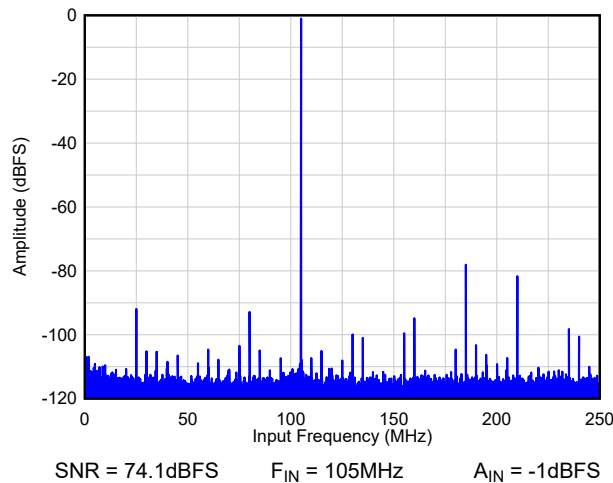
图 8-71. FFT - 无 AVG
