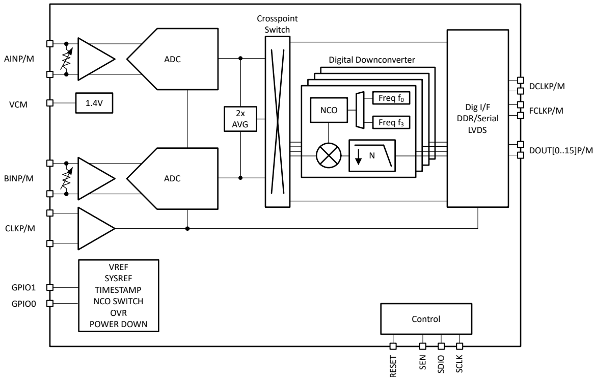
图 8-1. 方框图
