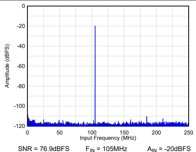
图 8-74. FFT - 2x AVG
