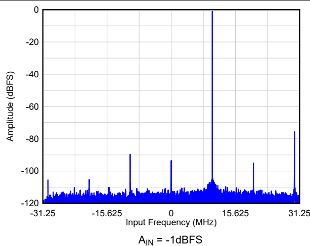
图 9-6. FFT3 : /8 抽取
