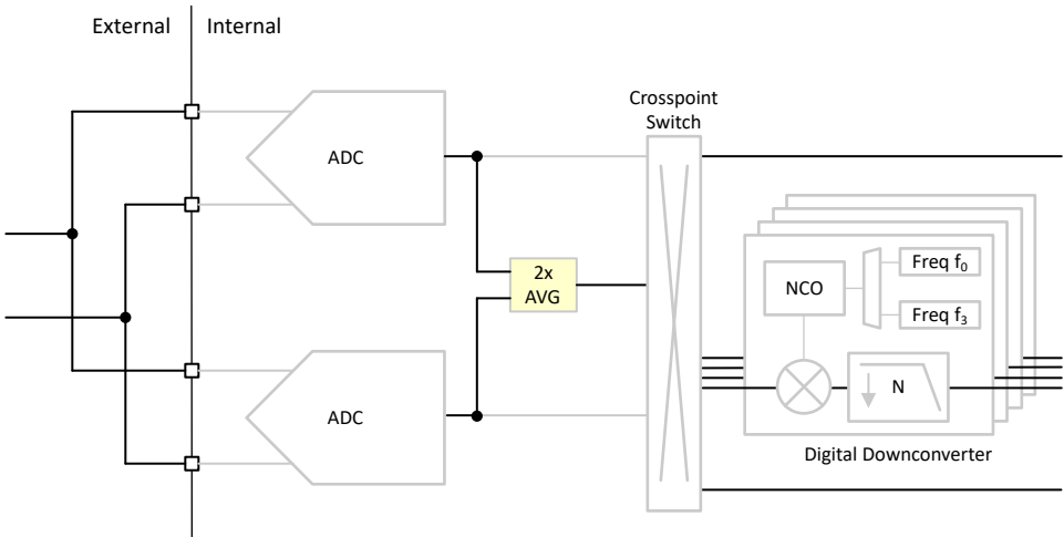
图 8-70. 数字通道平均示意图
