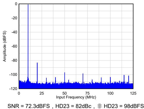
图 6-5. F_{IN} = 240\text{MHz} 时的单音 FFT
