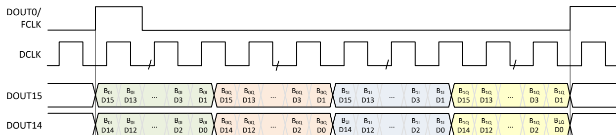
图 8-58. 示例 3 的 SLVDS 帧组装
