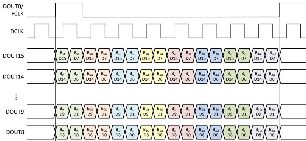
图 8-59. 示例 4 的 SLVDS 帧组装
