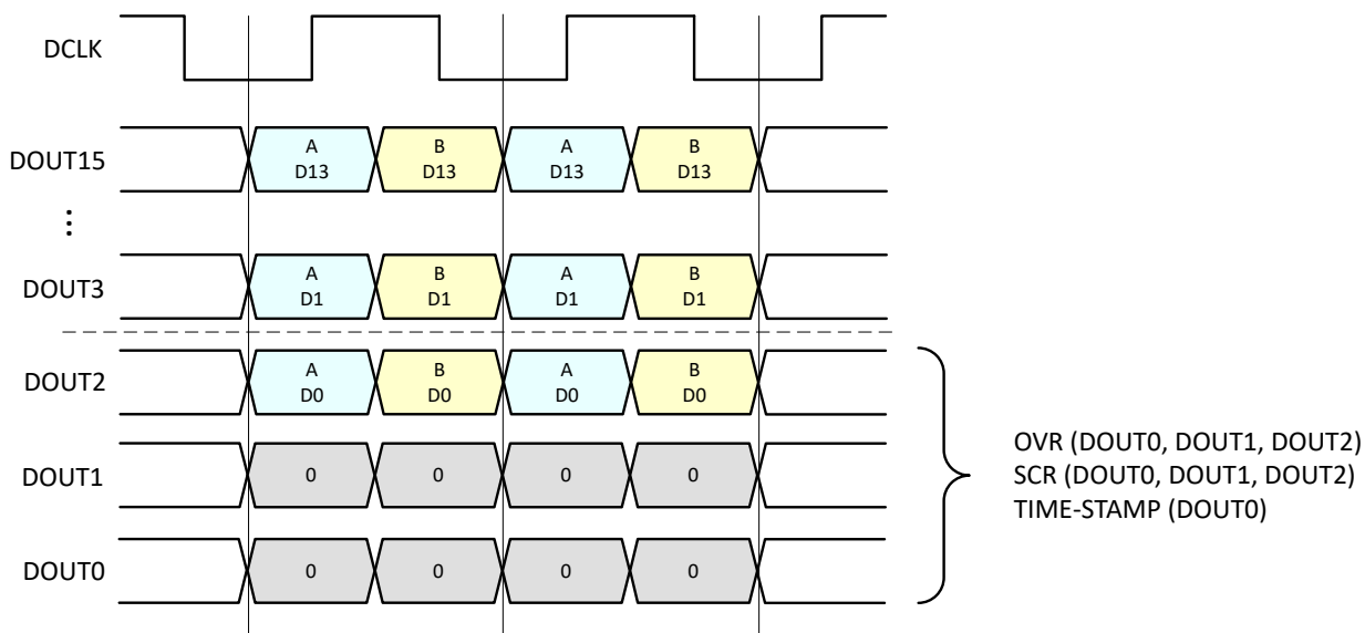
图 8-55. DDR LVDS 模式下的输出数据格式
