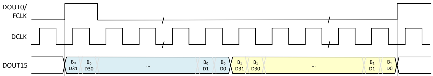
图 8-57. 示例 2 的 SLVDS 帧组装
