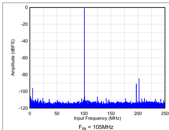
图 8-68. FFT : 正常模式
