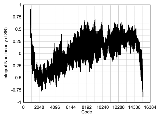
图 6-52. INL
