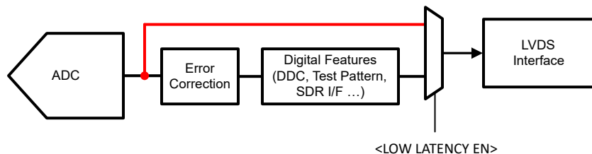
图 8-67. 低延迟模式
