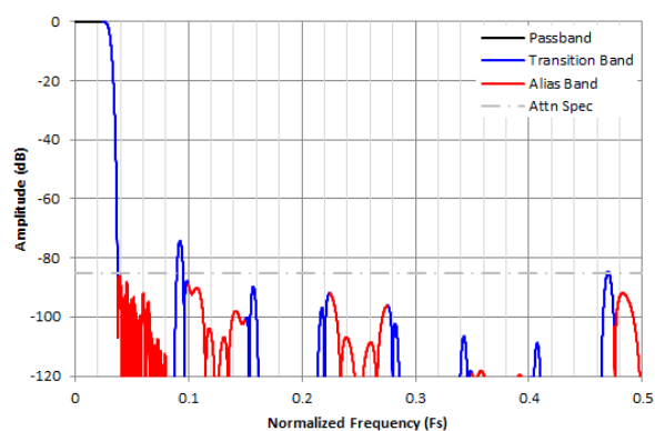
图 8-29. /16 复数抽取滤波器响应
