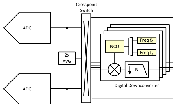
图 8-53. NCO 方框图
