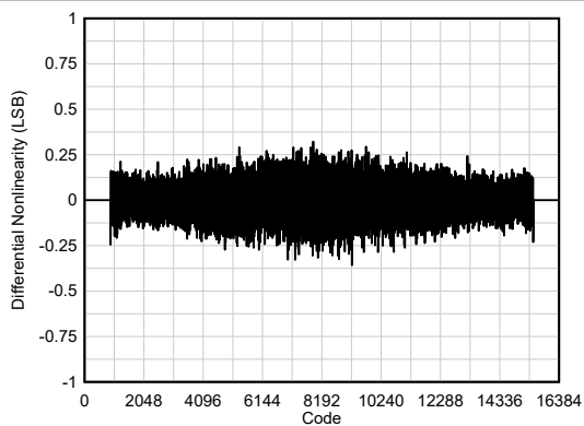
图 6-51. DNL
