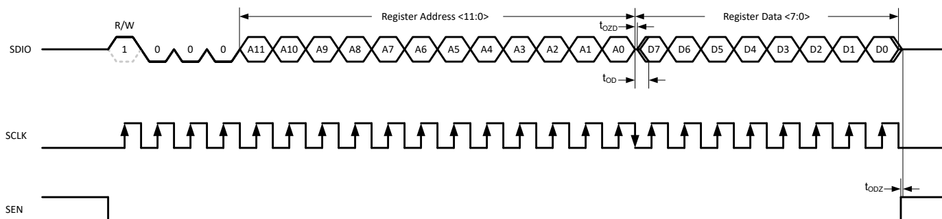
图 8-76. 串行寄存器读取时序图
