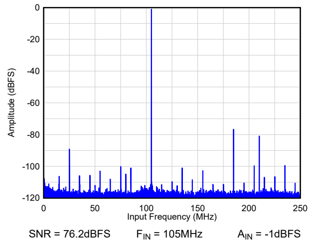
图 8-72. FFT - 2x AVG
