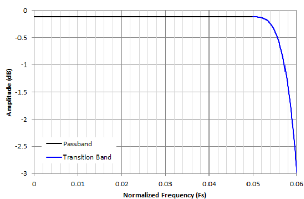
图 8-28. /8 抽取通带纹波响应
