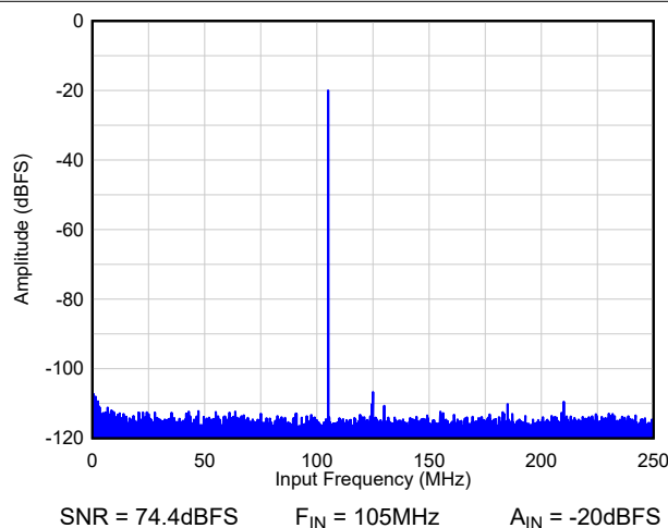
图 8-73. FFT - 无 AVG
