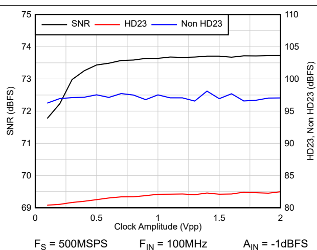
图 9-3. SNR 与时钟振幅间的关系
