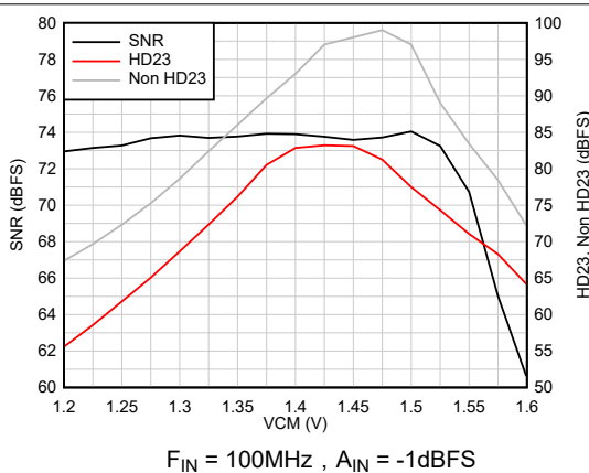
图 6-21. 交流性能与 VCM 间的关系
