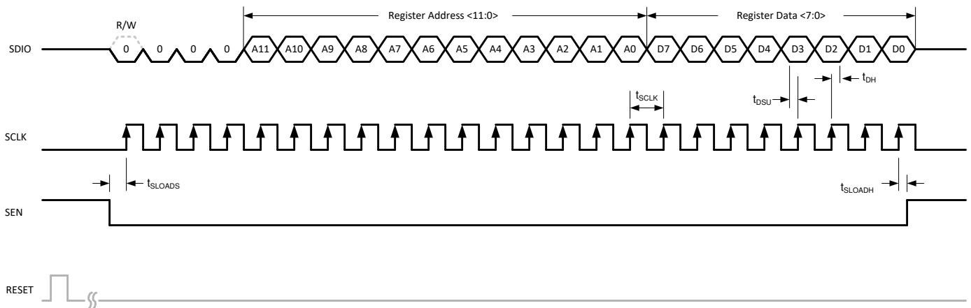
图 8-75. 串行寄存器写入时序图
