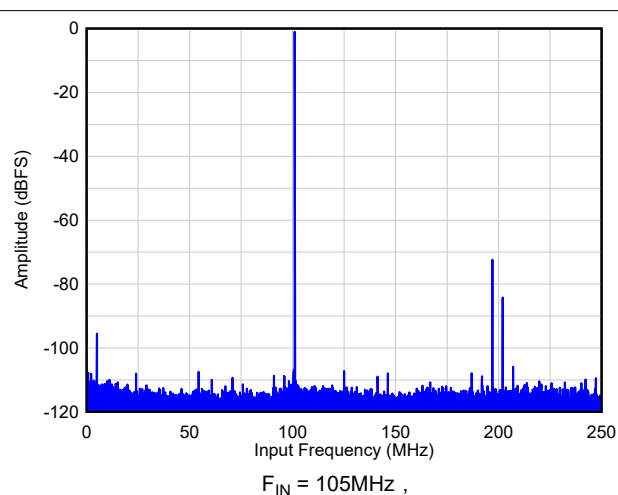
图 8-69. FFT : 低延迟模式
