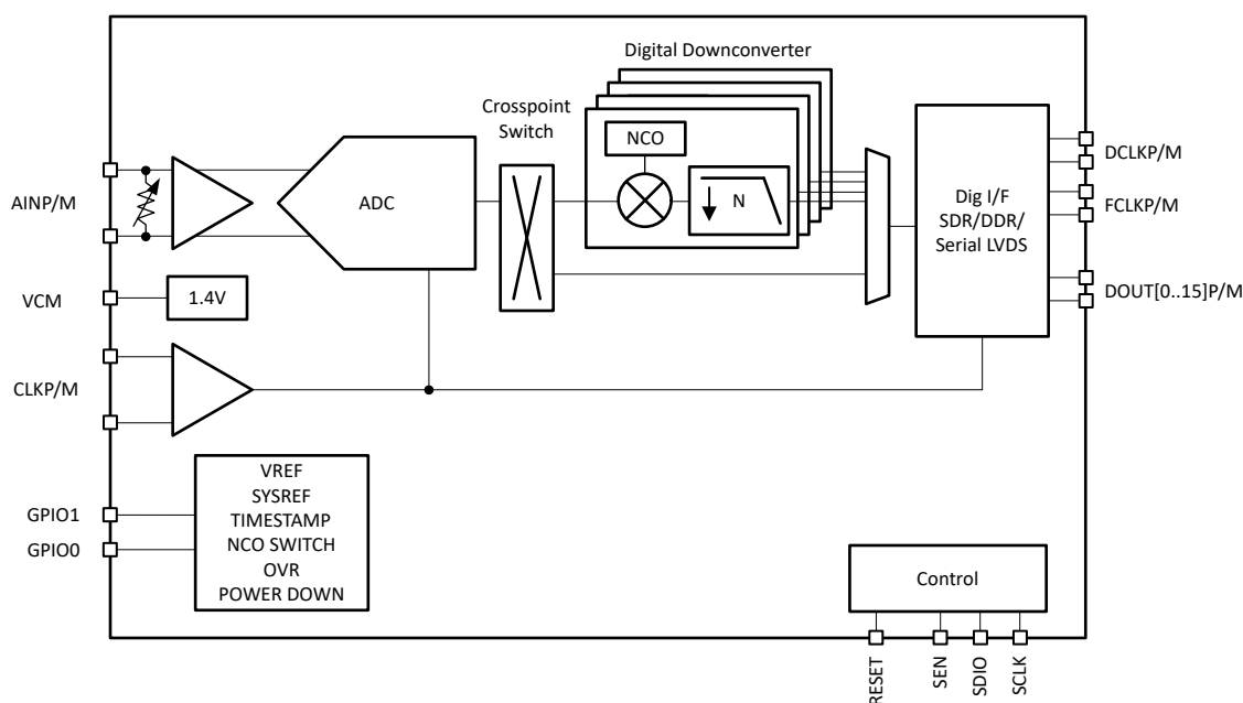
图 8-1. 方框图
