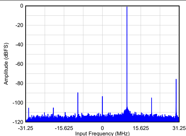
图 9-6. FFT3 : /8 抽取, A_{IN} = -1\text{dBFS}
