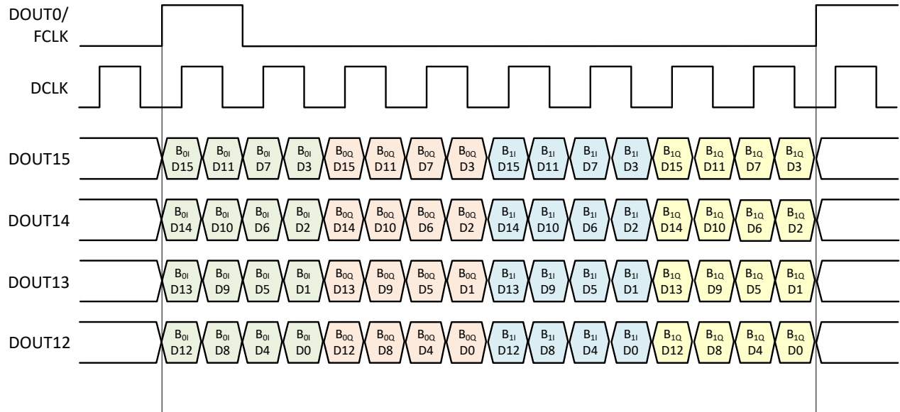
图 8-60. 示例 3 的 SLVDS 帧组装
