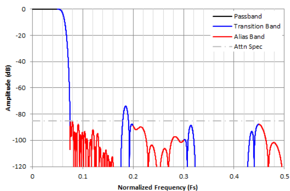
图 8-28. /8 复数抽取滤波器响应
