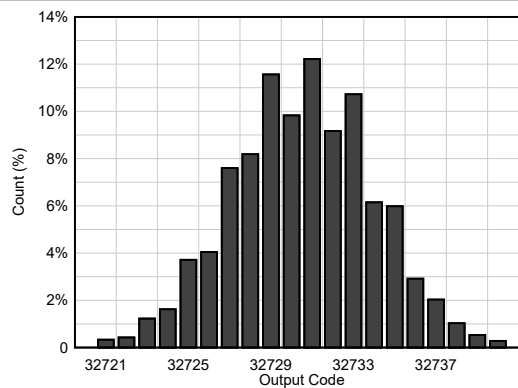
图 6-52. 直流偏移直方图
