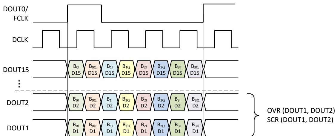
图 8-62. 输出数据替代：16 条 SLVDS 信道
