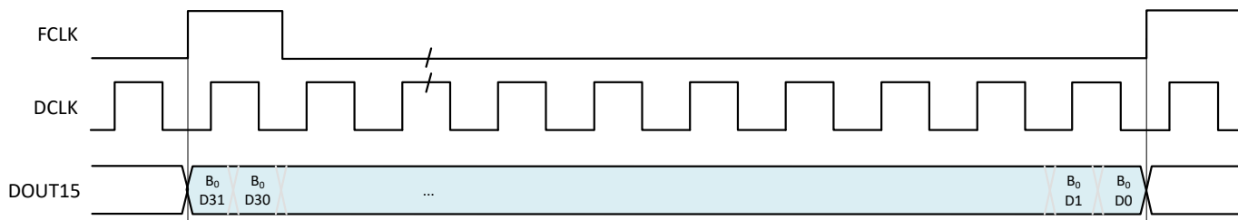
图 8-59. 示例 2 的 SLVDS 帧组装
