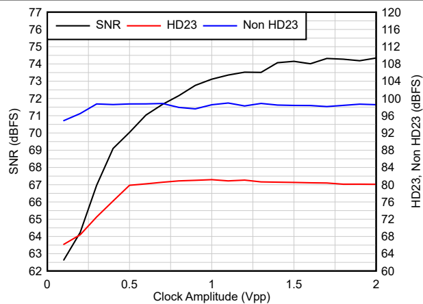
图 8-14. 交流与时钟振幅间的关系
