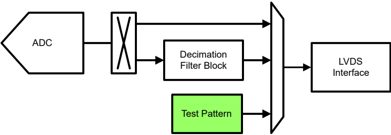
图 8-67. 测试图形发生器
