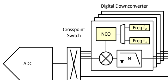
图 8-54. NCO 方框图
