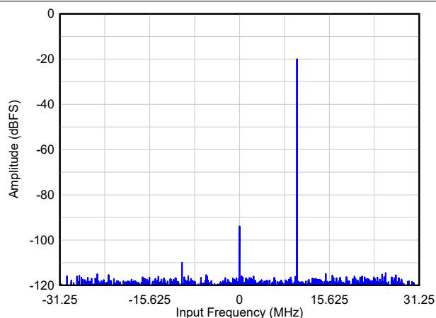
图 9-7. FFT4 : /8 抽取, A_{IN} = -20\text{dBFS}
