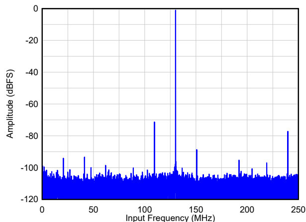
图 9-4. FFT1 : DDC 旁路, A_{IN} = -1\text{dBFS}
