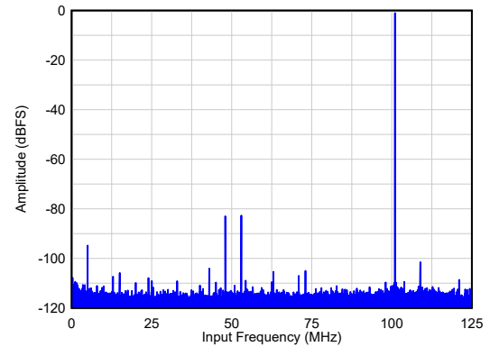
图 6-2. F_{IN} = 101\text{MHz} 时的单音 FFT
