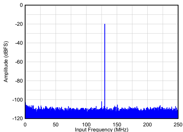
图 9-5. FFT2 : DDC 旁路, A_{IN} = -20\text{dBFS}
