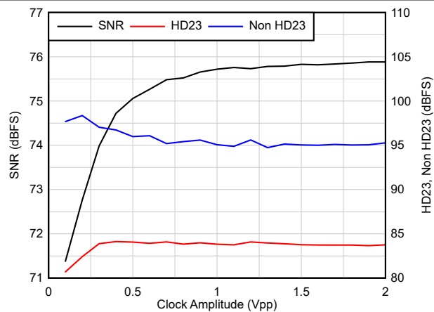
图 8-13. 交流与时钟振幅间的关系
