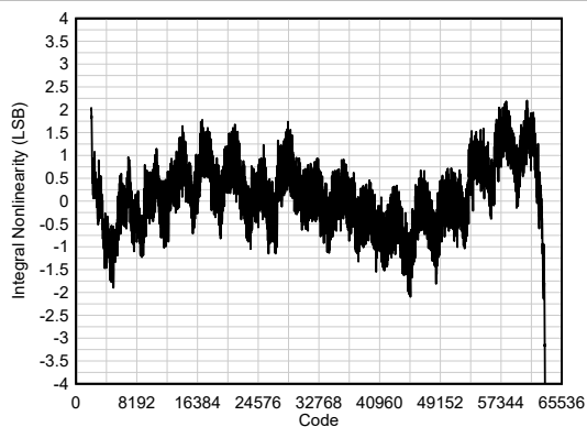
图 6-51. INL
