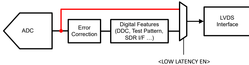
图 8-68. 低延迟模式
