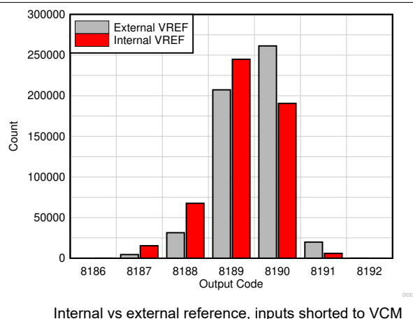
图 6-19. DC Histogram
