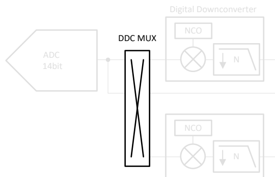
图 8-14. DDC MUX
