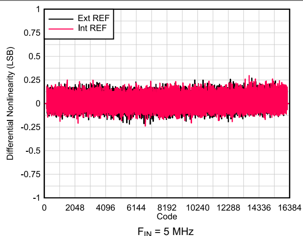
图 6-56. DNL vs Code
