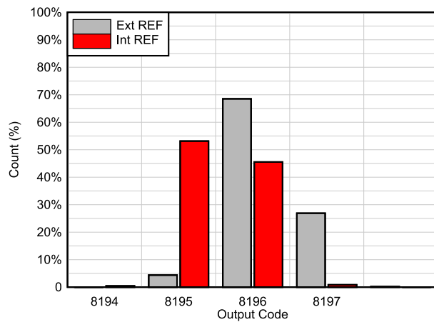
图 6-34. DC Histogram
