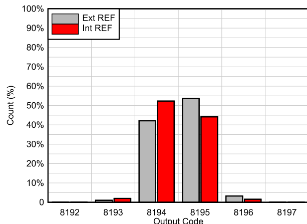
图 6-57. DC Histogram
