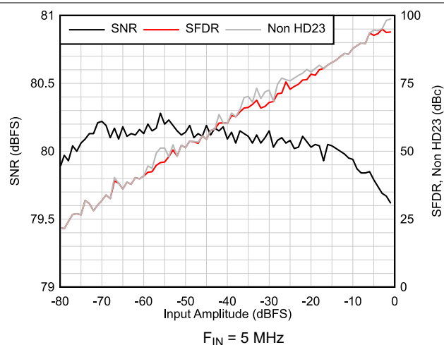
图 6-27. AC Performance vs Input Amplitude
