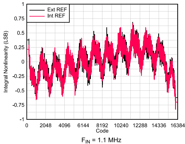
图 6-32. INL vs Code
