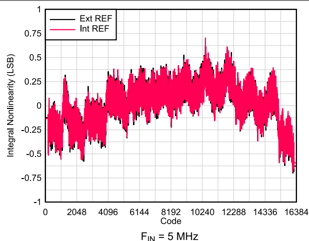
图 6-55. INL vs Code
