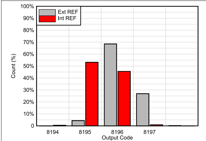
图 6-34. DC Histogram
