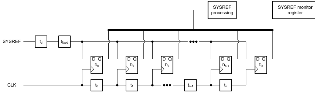
图 7-10. SYSREF 检测电路
