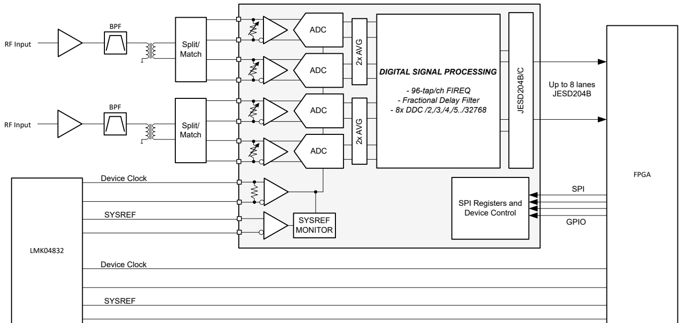
图 8-1. 宽带射频采样接收器
