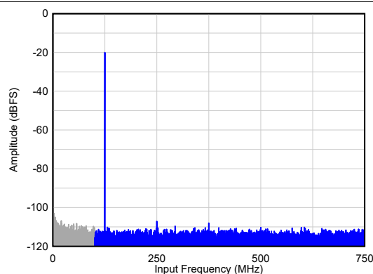
图 7-40. 单音 FFT，正常模式
