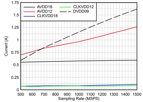
图 5-26. 电流与采样率间的关系
