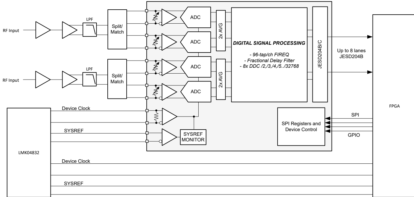
图 8-8. 时间域数字转换器
