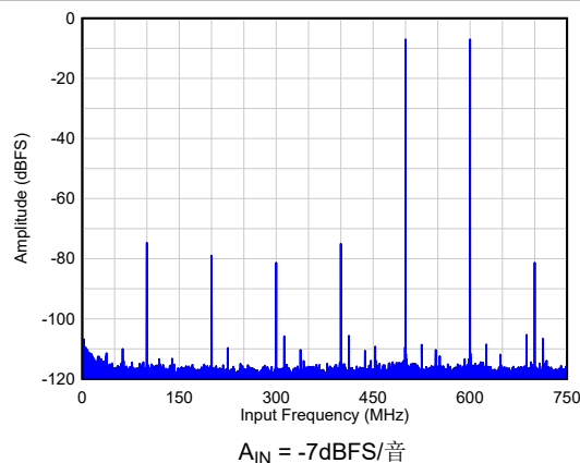
图 5-8. F_{IN} = 900\text{MHz}/1000\text{MHz} 时的双音 FFT
