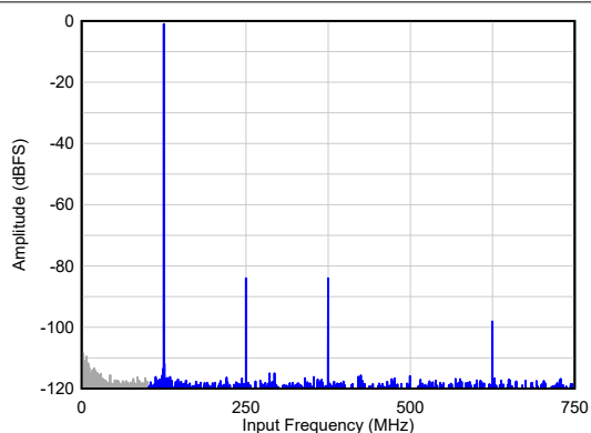
图 7-41. 单音 FFT，对 2 次结果取平均值模式
