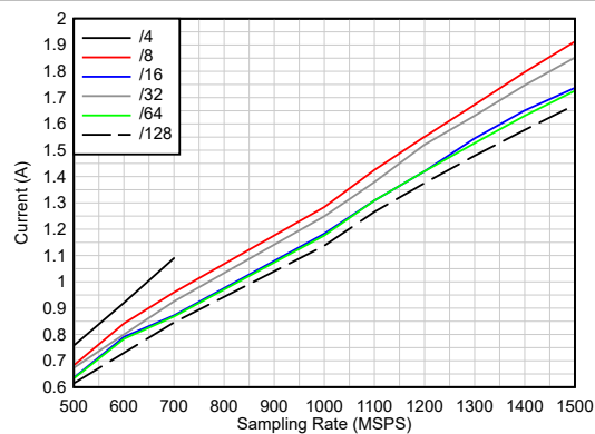
图 5-32. DVDD09 电流与抽取间的关系
