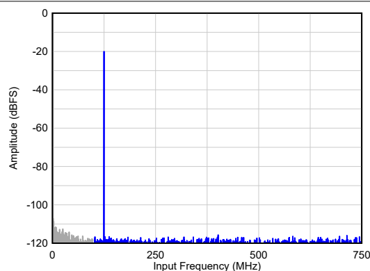
图 7-42. 单音 FFT，对 2 次结果取平均值模式
