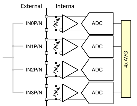
图 7-38. 工作模式：对 4 次结果取平均值
