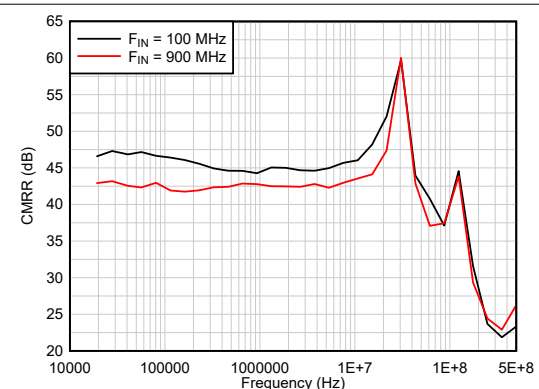
图 5-24. CMRR
