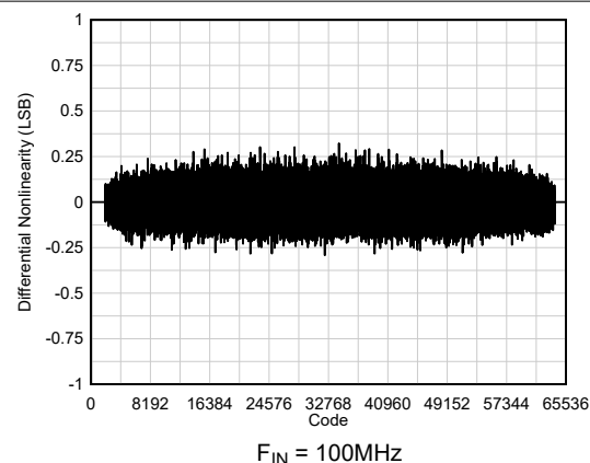
图 5-22. DNL 与代码间的关系
