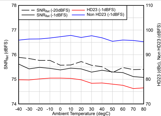
图 5-20. 交流性能与温度间的关系
