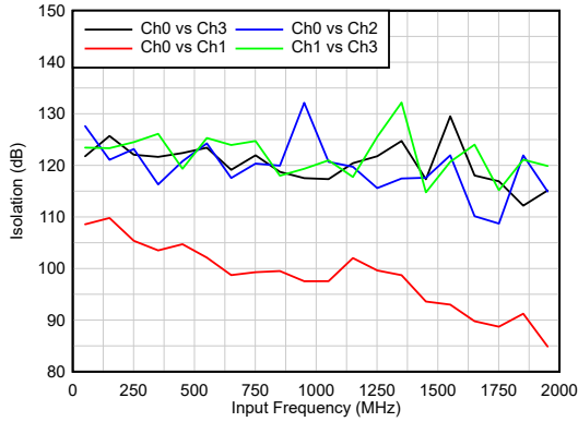
图 5-25. 通道隔离
