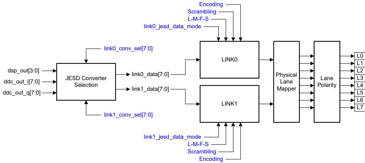
图 7-34. JESD204 方框图
