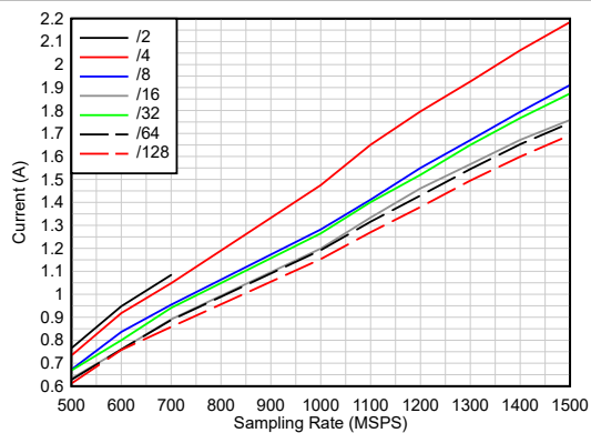
图 5-31. DVDD09 电流与抽取间的关系
