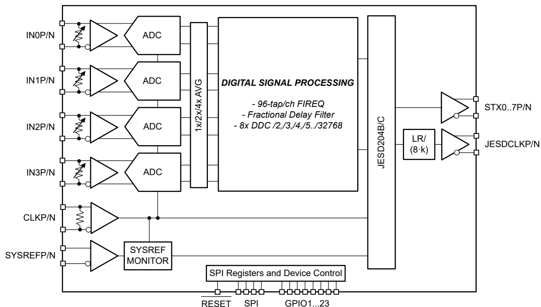
方框图
