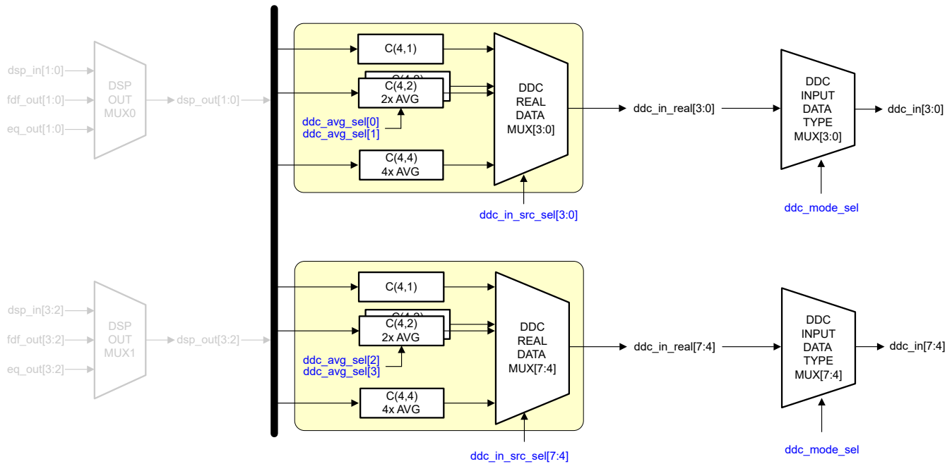
图 7-22. DDC 输入数据多路复用
