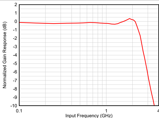
图 7-4. 输入带宽图
