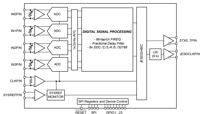
方框图
