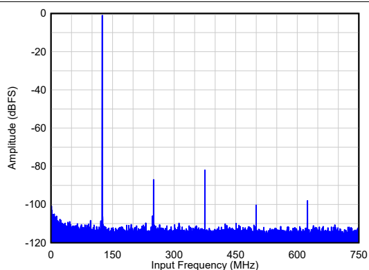
图 7-39. 单音 FFT，正常模式
