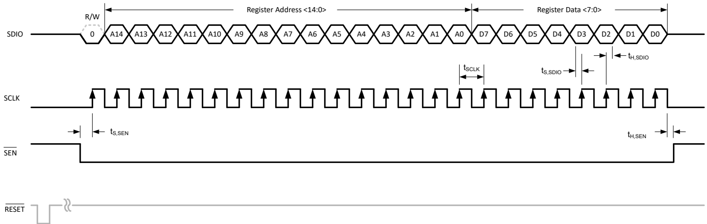
图 7-45. 串行寄存器写入时序图
