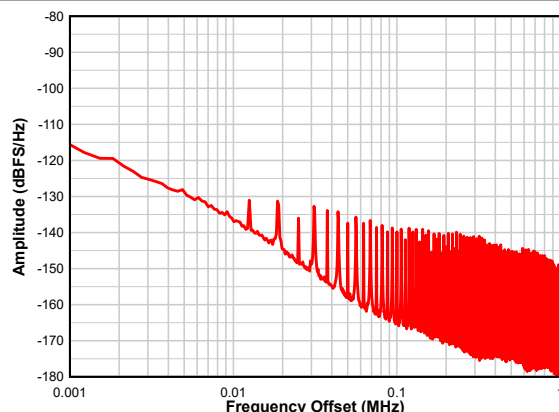
图 6-8. Dither Close-Up
