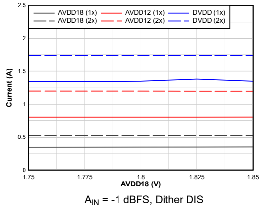
图 6-51. Current vs AVDD18
