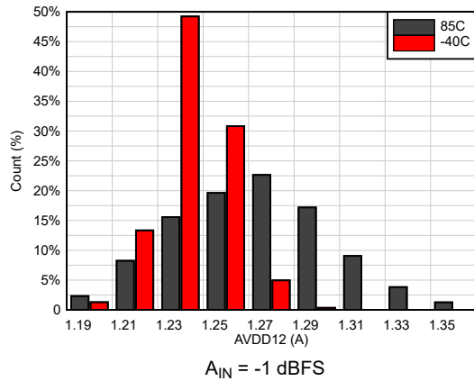
图 6-55. AVDD12 Distribution
