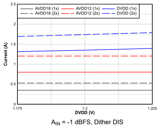
图 6-53. Current vs DVDD
