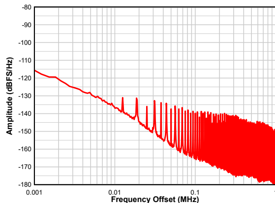
图 7-6. Dither Close-Up
