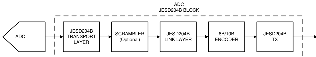
图 7-38. JESD204B Block Diagram
