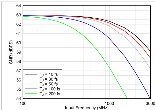
图 8-2. SNR vs T_{Jitter} vs F_{IN} (1x AVG)
