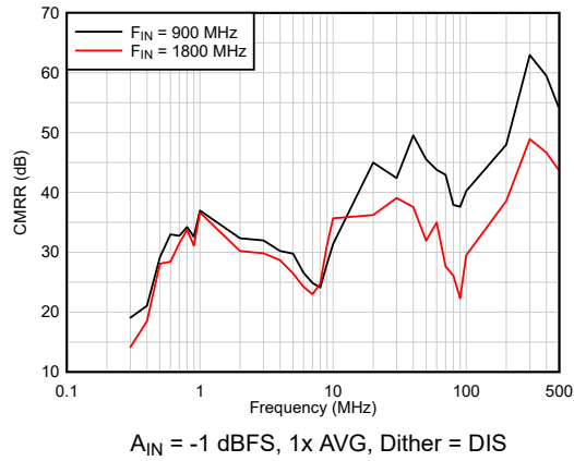
图 6-43. CMRR
