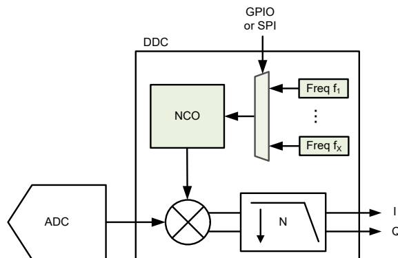
图 7-38. NCO Block Diagram
