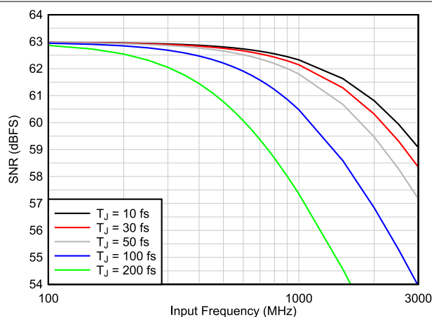
图 8-2. SNR vs T_{Jitter} vs F_{IN} (1x AVG)
