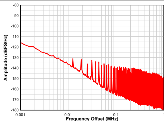
图 7-6. Dither Close-Up
