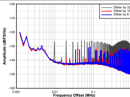
图 7-7. Dither vs Dither Divider Setting
