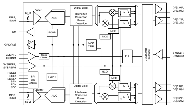
简化框图
