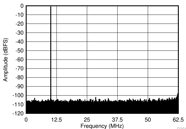
f_S = 125\text{MSPS} 且 f_{IN} = 10\text{MHz} 时的性能 ( \text{SNR} = 70.6\text{dBFS} ， \text{SFDR} = 100\text{dBc} )
