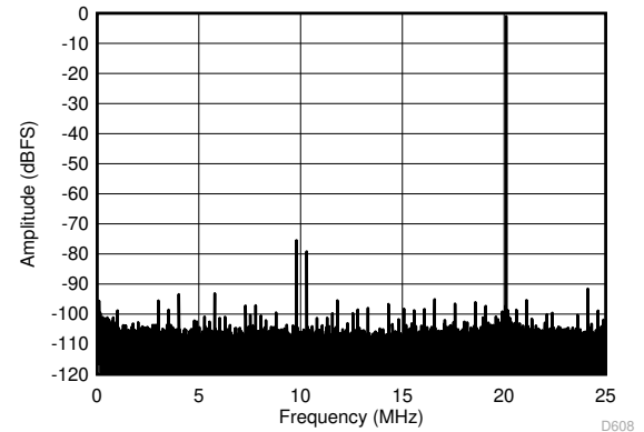
图 6-36. FFT for 170-MHz Input Signal (Dither Off)
