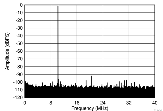
图 6-64. FFT for 70-MHz Input Signal (Dither Off)
