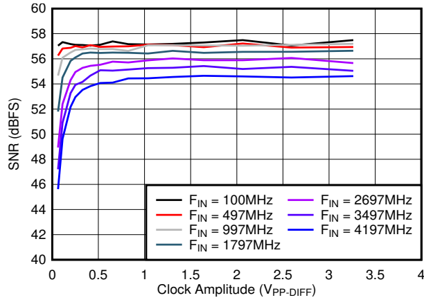
图 5-37. SNR vs A_CLK
