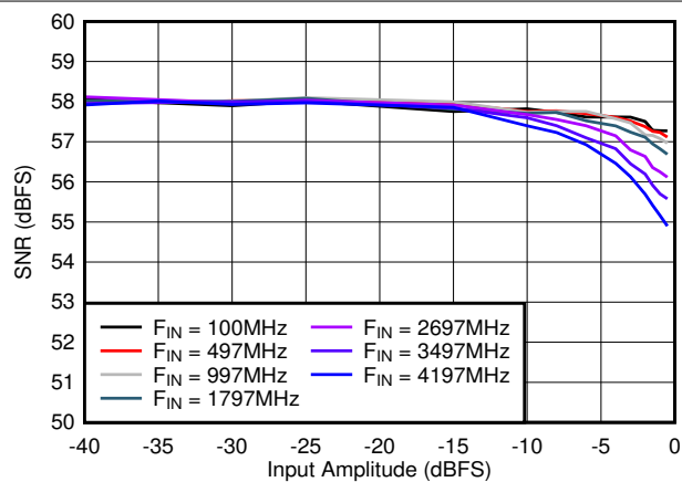
图 5-33. SNR vs A_{IN}
