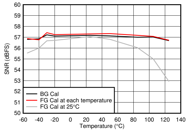
图 5-64. SNR vs Temperature
