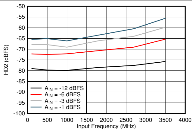
图 5-21. HD2 vs Input Frequency
