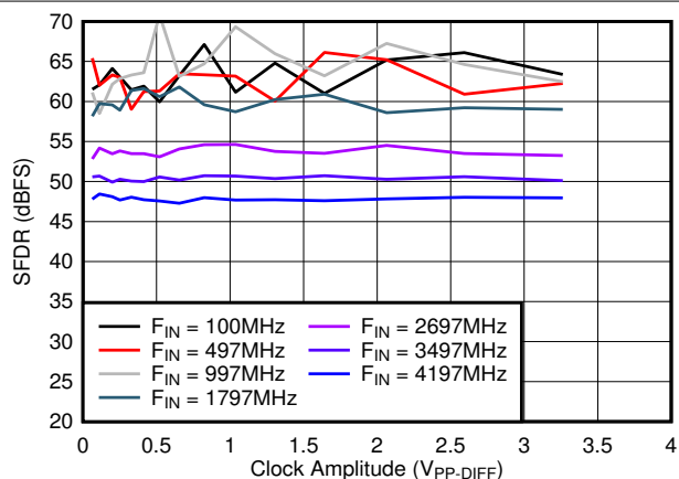
图 5-36. SFDR vs A_{CLK}
