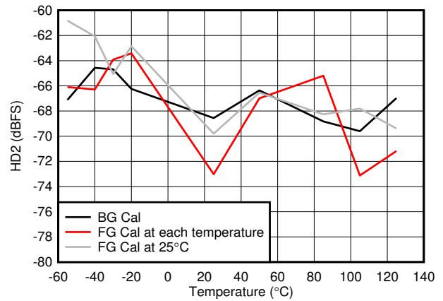
图 5-66. HD2 vs Temperature
