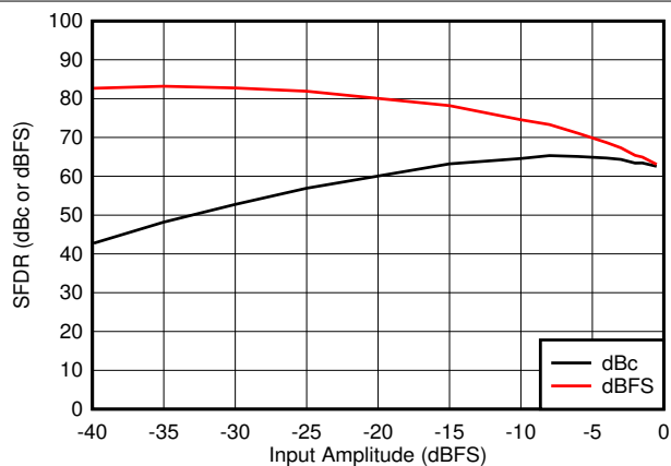
图 5-34. SFDR vs A_{IN}
