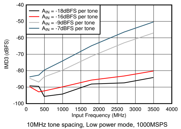
图 5-76. IMD3 vs F_{IN}
