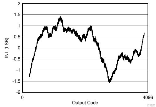
图 5-2. INL vs Code
