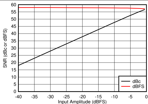
图 5-35. SNR vs A_{IN}
