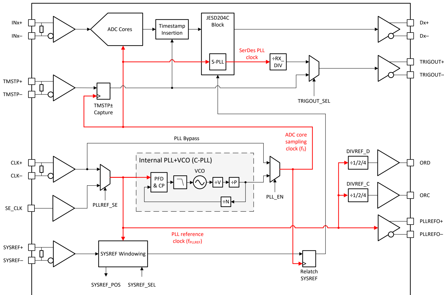
图 6-5. Clocking Subsystem
