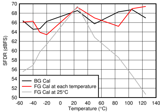
图 5-65. SFDR vs Temperature
