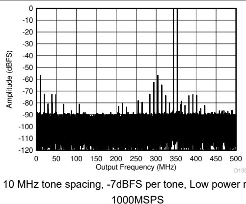
图 5-72. Two Tone FFT at 348 MHz
