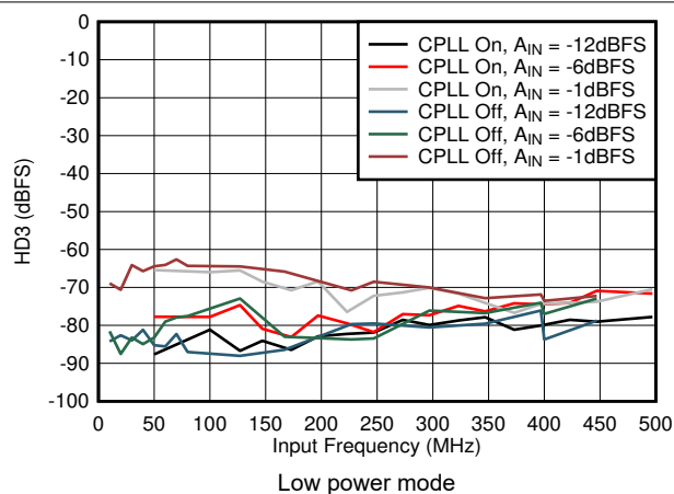
图 5-59. HD3 vs A_{IN} and C-PLL
