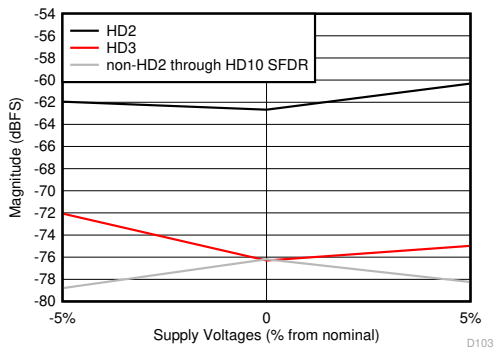
图 5-61. HD2、HD3 和最差非 HD 杂散与电源电压间的关系
