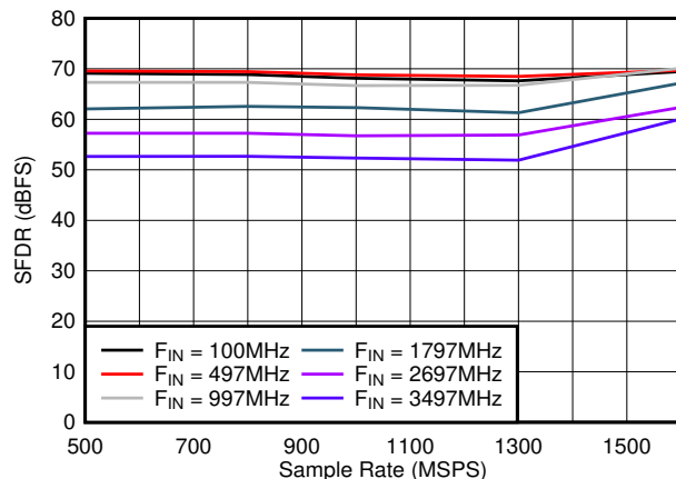
图 5-23. SFDR 与采样率间的关系
