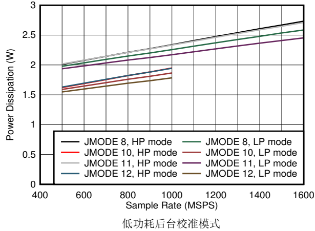
图 5-81. 四通道, 功率耗散与 F_S 以及 JMODES 8 - 12 间的关系
