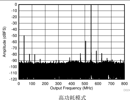
图 5-11. 3797MHz 和 -1dBFS 条件下的单频 FFT
