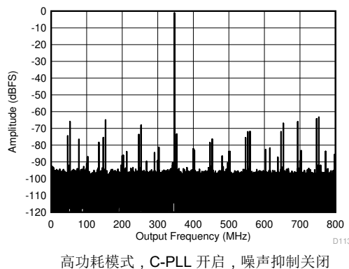
图 5-6. 347MHz 和 -1dBFS 条件下的单频 FFT
