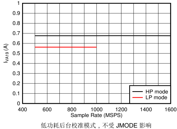
图 5-83. 四通道, I_{VA19} 与 F_S 间的关系
