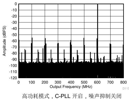
图 5-9. 997MHz 和 -1dBFS 条件下的单频 FFT
