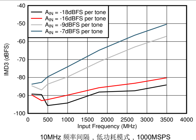
图 5-76. IMD3 与 F_{IN} 间的关系
