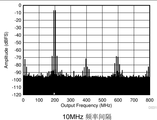
图 5-70. 1798MHz 时的双音 FFT
