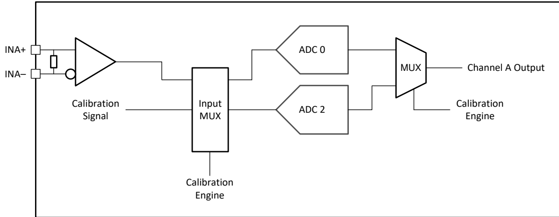
图 6-15. 单通道校准系统方框图
