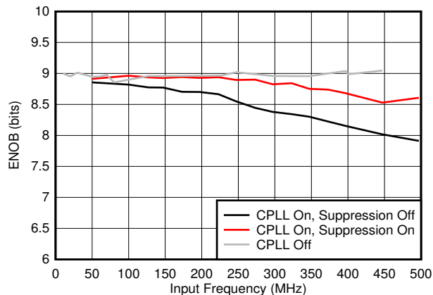
图 5-47. ENOB 与 F_{IN} 以及 C-PLL 模式间的关系
