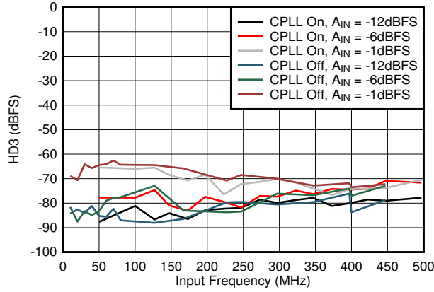
图 5-59. HD3 与 A_{IN} 以及 C-PLL 间的关系
