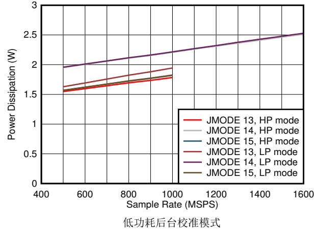
图 5-82. 四通道, 功率耗散与 F_S 以及 JMODES 13 - 15 间的关系
