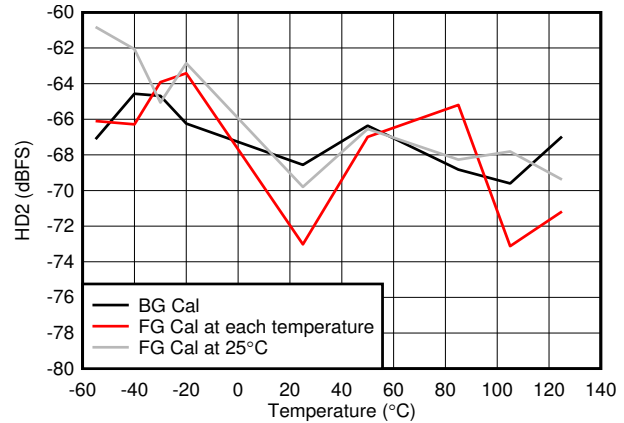
图 5-66. HD2 与温度间的关系
