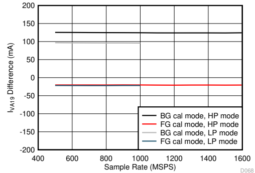
图 5-112. 四通道, 校准模式下的 I_{VA19} 变化
