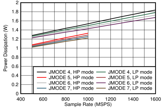
图 5-90. 双通道, 功率耗散与 F_S 以及 JMODE 4 - 7 间的关系
