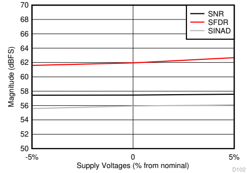
图 5-62. SNR、SFDR 和 SINAD 与电源电压间的关系
