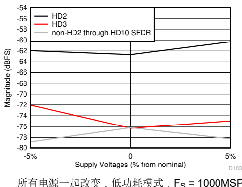
图 5-63. HD2、HD3 和最差非 HD 杂散与电源电压间的关系
