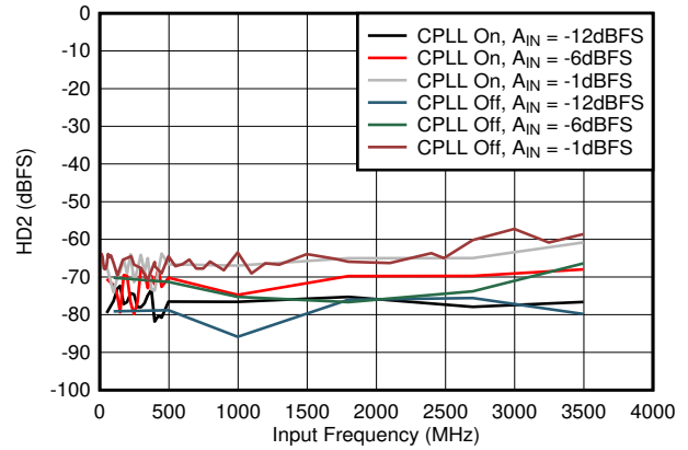
图 5-52. HD2 与 A_{IN} 以及 C-PLL 间的关系
