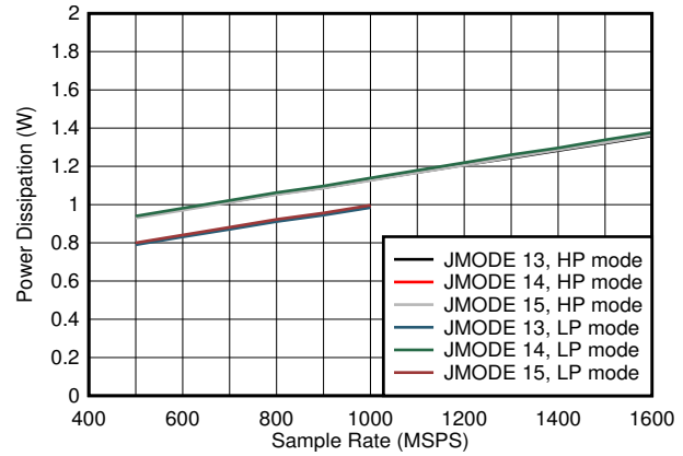
图 5-102. 单通道, 功率耗散与 F_S 和 JMODE 13 - 15 间的关系
