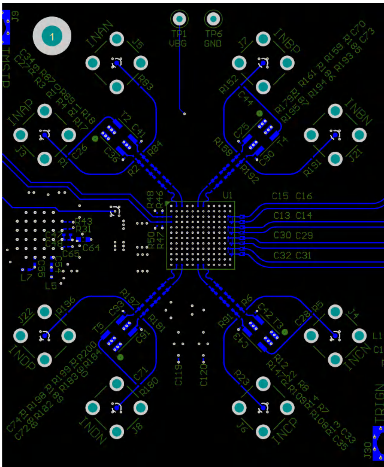
图 7-5. 顶层布线：模拟输入 (INA±、INB±、INC±、IND±)、TMSTP± 和 D[3:0]± 布线
