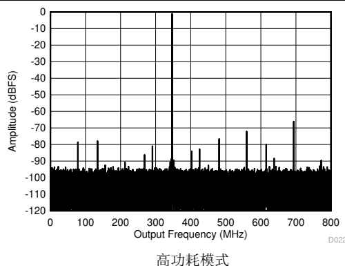
图 5-4. 347MHz 和 -1dBFS 条件下的单频 FFT
