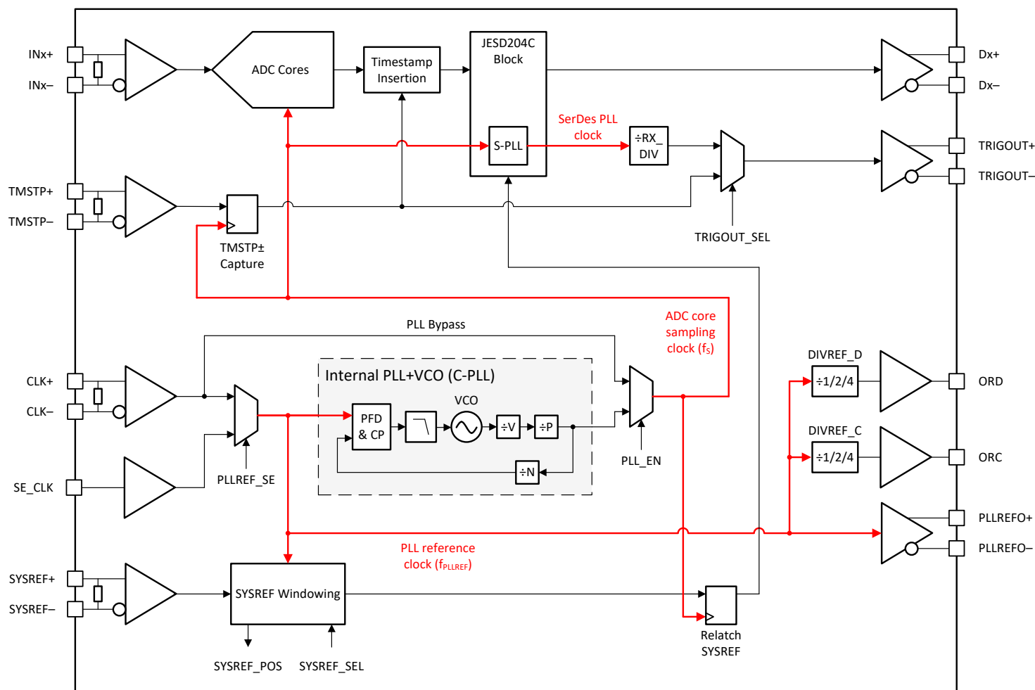
图 6-3. Clocking Subsystem
