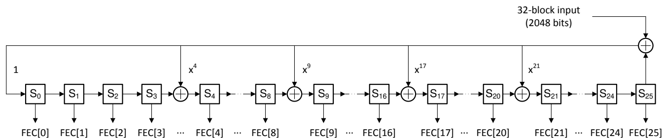
图 6-8. FEC Parity Bit Generator
