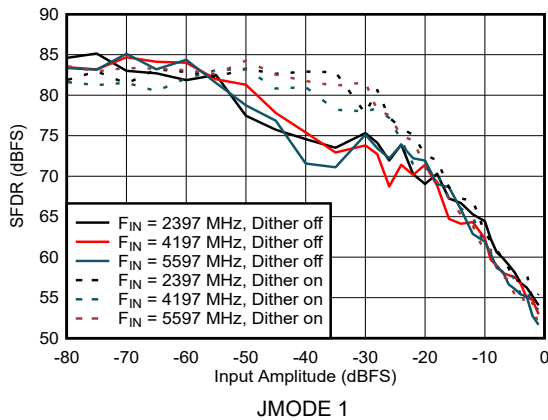
图 5-15. DES Mode: SFDR vs Input Amplitude
