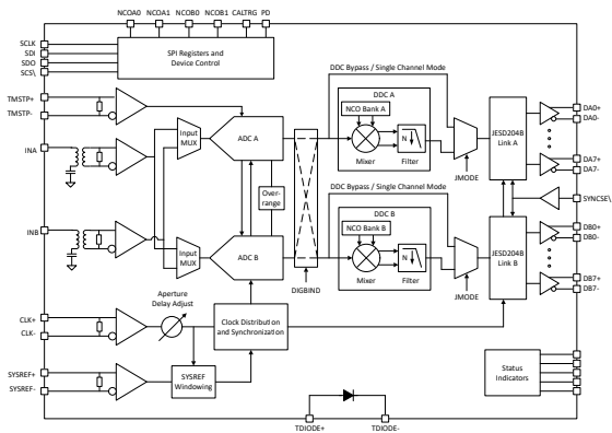
ADC12DJ5200SE 方框图
