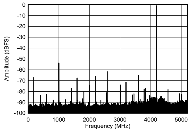
图 7-3. FFT for 4197 MHz Input Signal, 10.4 GSPS, JMODE1
