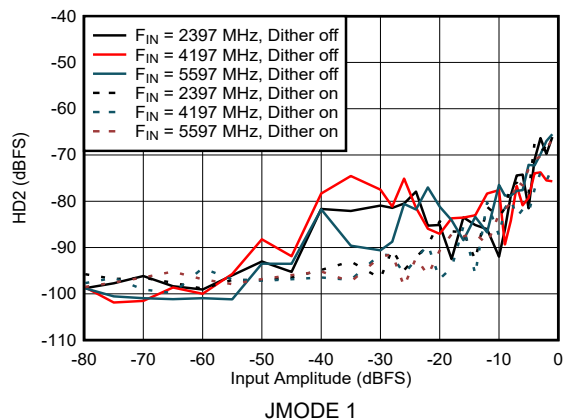
图 5-17. DES Mode: HD2 vs Input Amplitude
