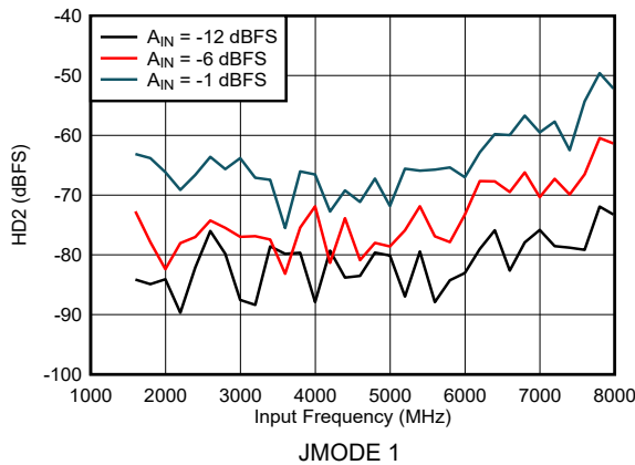
图 5-11. DES Mode: HD2 vs Input Frequency
