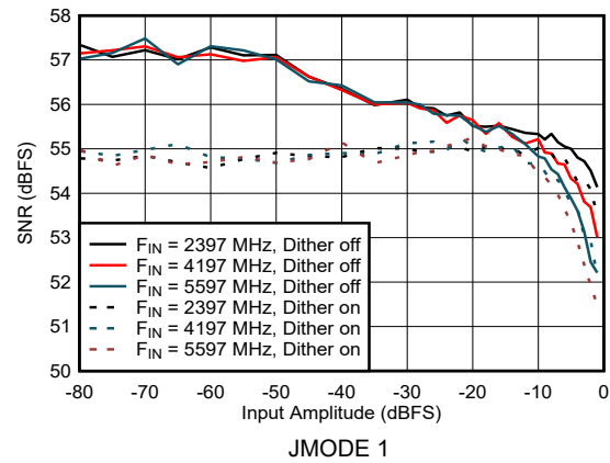
图 5-14. DES Mode: SNR vs Input Amplitude
