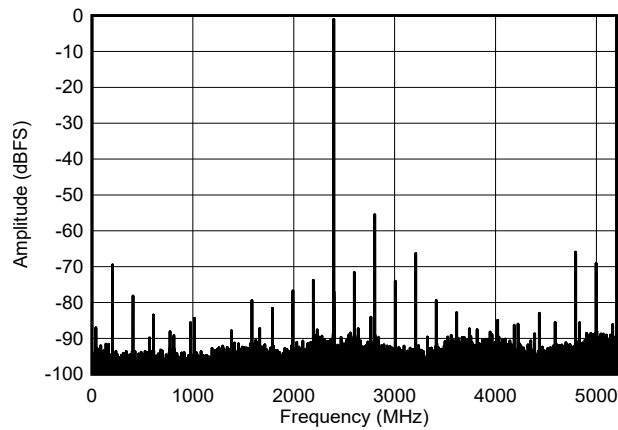
图 7-2. FFT for 2397 MHz Input Signal, 10.4 GSPS, JMODE1
