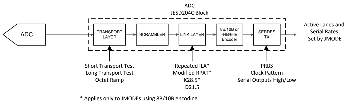
图 6-25. Test Mode Insertion Points
