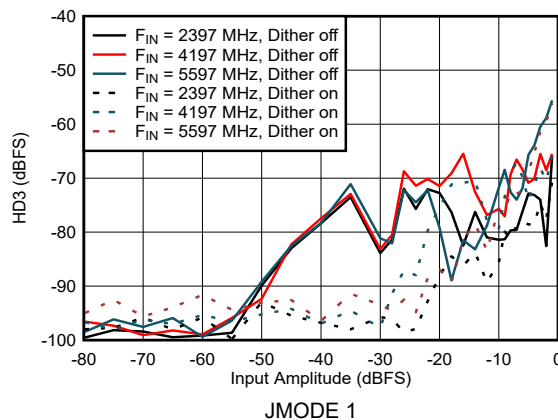
图 5-18. DES Mode: HD3 vs Input Amplitude
