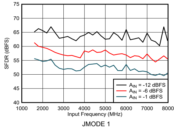
图 5-9. DES Mode: SFDR vs Input Frequency
