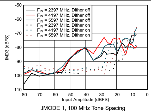
图 5-24. DES Mode: IMD3 vs Input Amplitude
