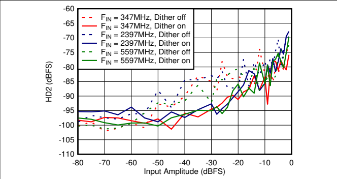
图 5-62. DES Mode: HD2 vs Input Amplitude and Dither
