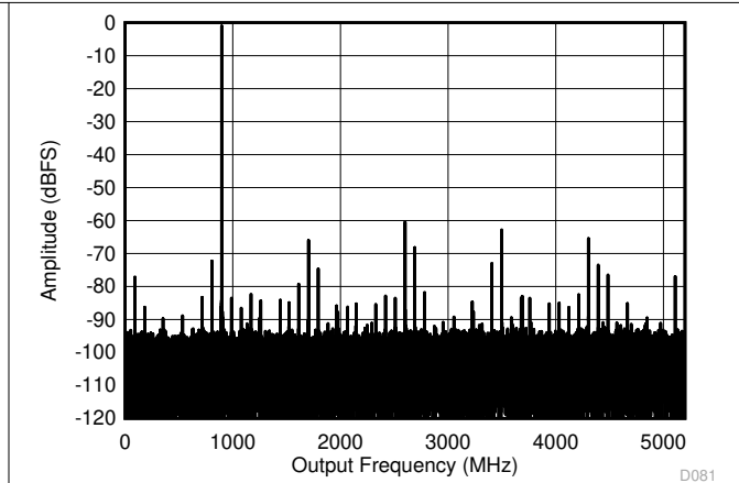
图 5-6. DES Mode: Single Tone FFT at 897 MHz
