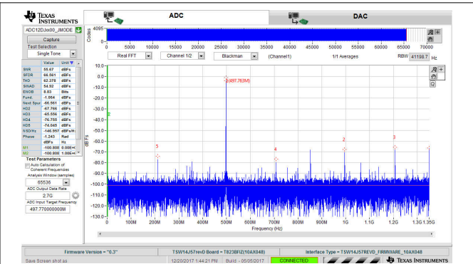
图 7-3. FFT for 497.77-MHz Input Signal, 2.7 GSPS, JMODE2
