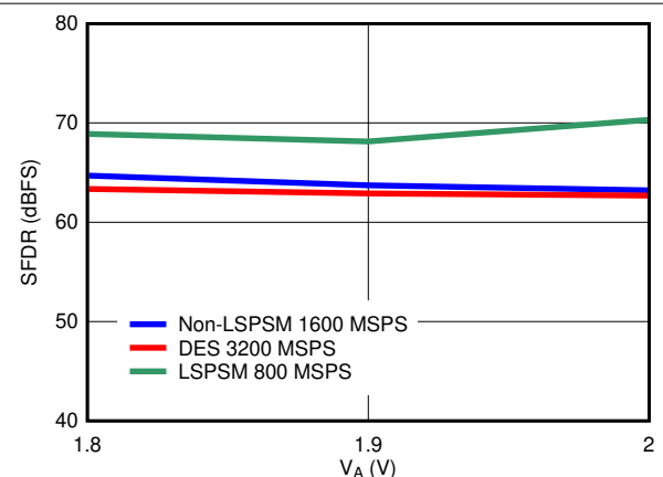
图 6-28. SFDR vs Supply Voltage
