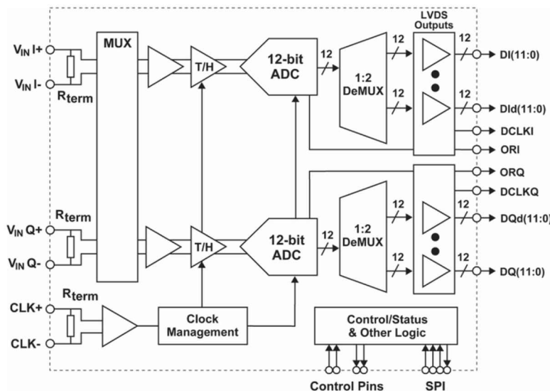
功能方框图
