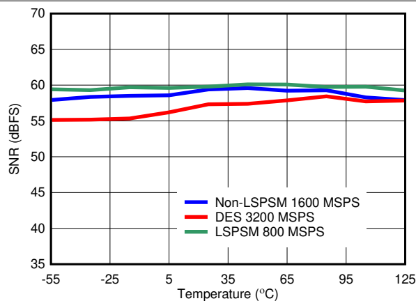
图 6-21. SNR vs Temperature
