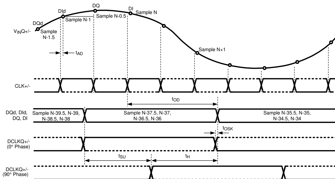
图 6-3. Clocking in Non-LSPSM, 1:4 Demux DES Mode*
