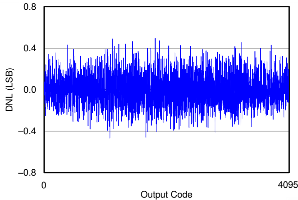
图 6-13. DNL vs Code
