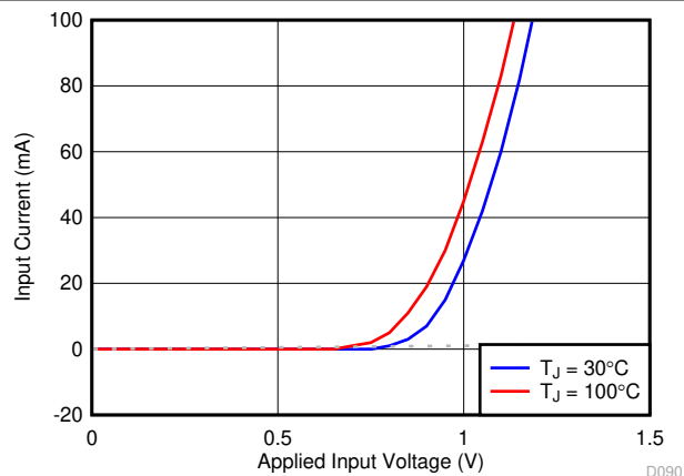
图 8-7. ESD Diode Current
