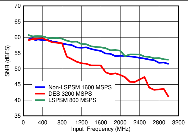
图 6-22. SNR vs Input Frequency
