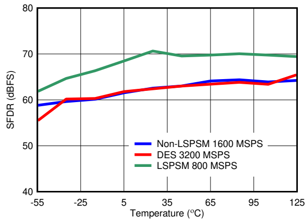
图 6-29. SFDR vs Temperature
