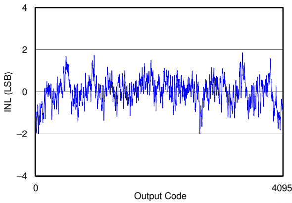
图 6-11. INL vs Code
