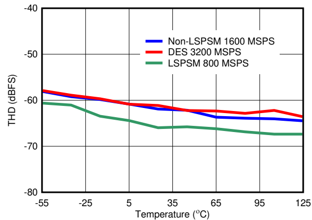
图 6-25. THD vs Temperature
