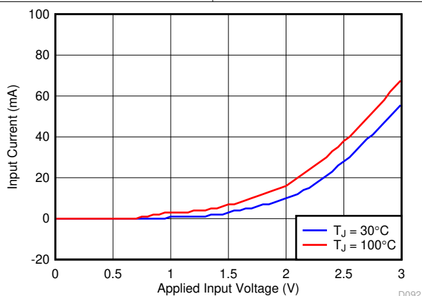
图 8-8. ESD Diode Current
