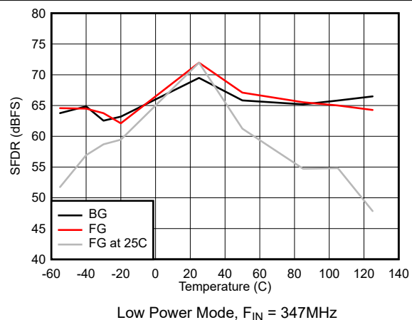
图 5-41. SFDR vs Temperature
