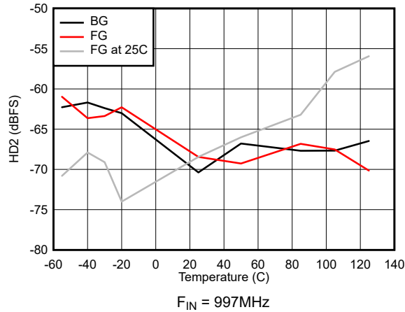
图 5-37. HD2 vs Temperature
