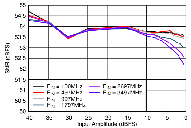
图 5-30. SNR vs Input Amplitude
