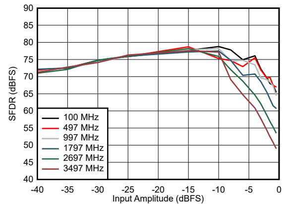
图 5-28. SFDR vs Input Amplitude
