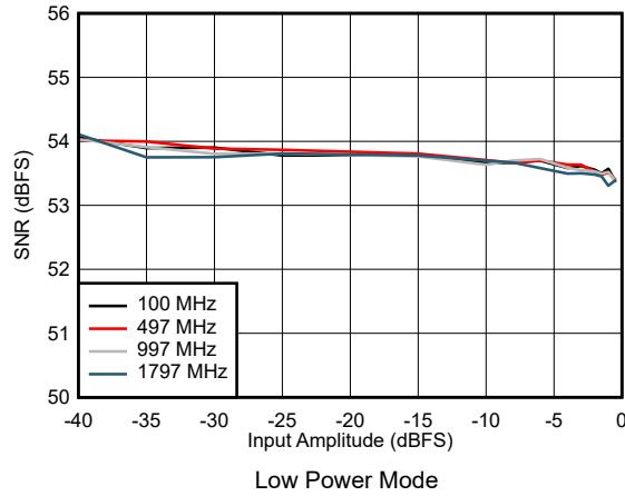
图 5-31. SNR vs Input Amplitude
