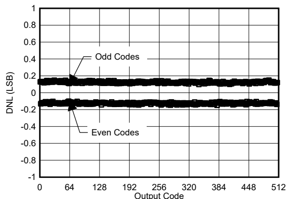
图 5-1. DNL vs Code
