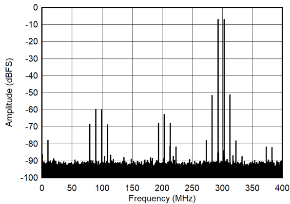
图 5-55. Dual Tone FFT at 2698 MHz
