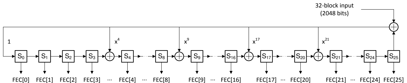
图 6-10. FEC Parity Bit Generator
