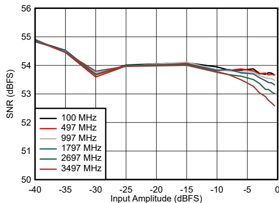
图 5-29. SNR vs Input Amplitude
