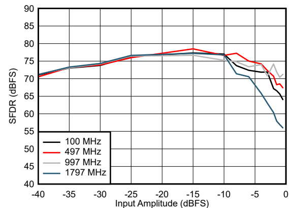
图 5-30. SFDR vs Input Amplitude
