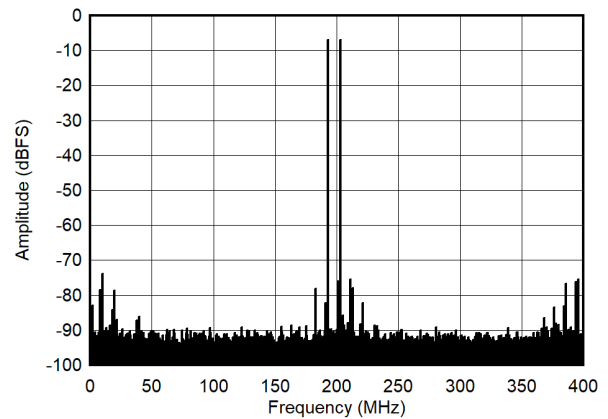
图 5-52. Dual Tone FFT at 998 MHz
