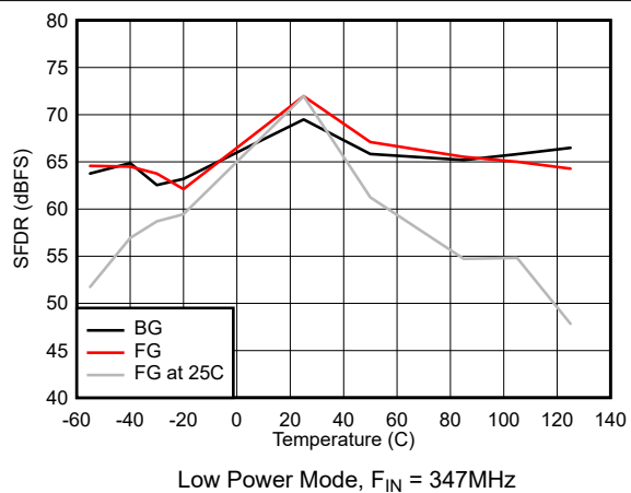
图 5-41. SFDR vs Temperature
