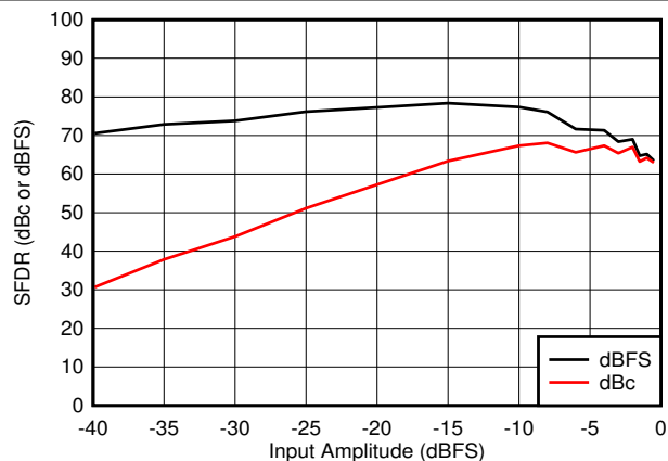
图 5-31. SFDR vs Input Amplitude
