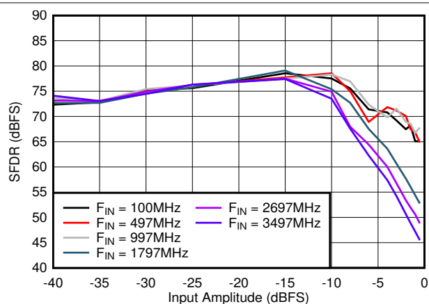
图 5-29. SFDR vs Input Amplitude
