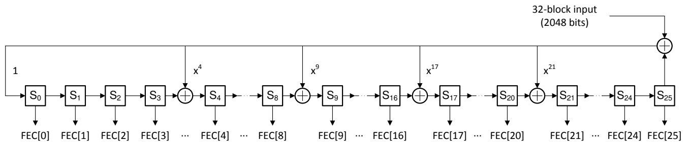
图 6-10. FEC Parity Bit Generator
