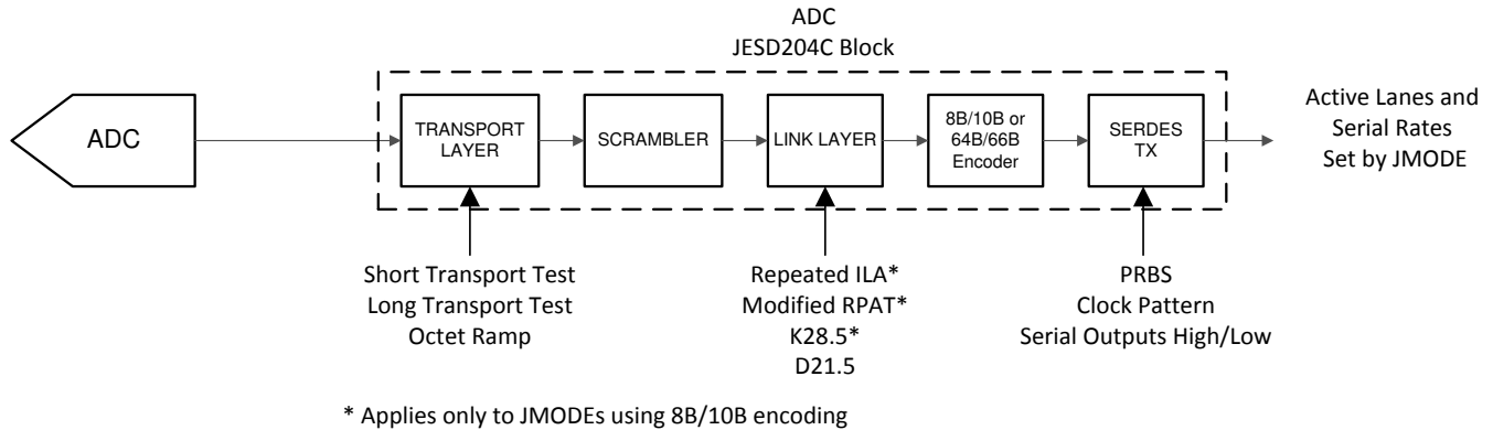
图 6-14. Test Mode Insertion Points
