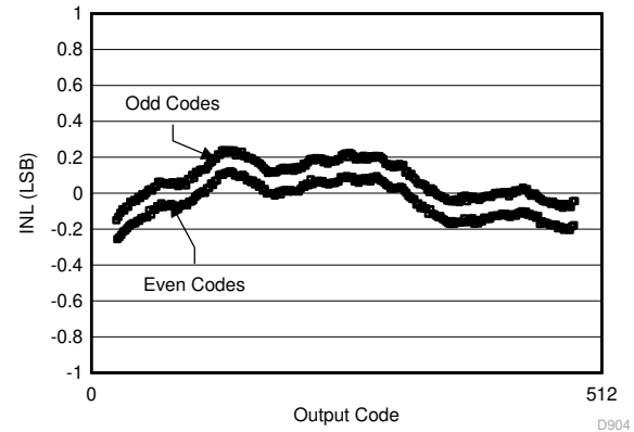
图 5-2. INL vs Code
