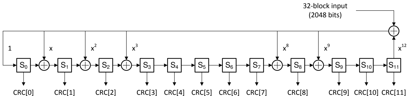
图 6-9. CRC-12 Parity Bit Generator
