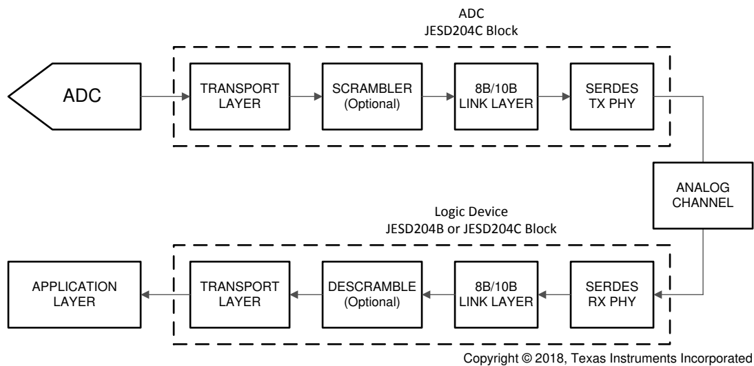
图 6-7. Simplified 8B/10B Encoded JESD204C Interface Diagram
