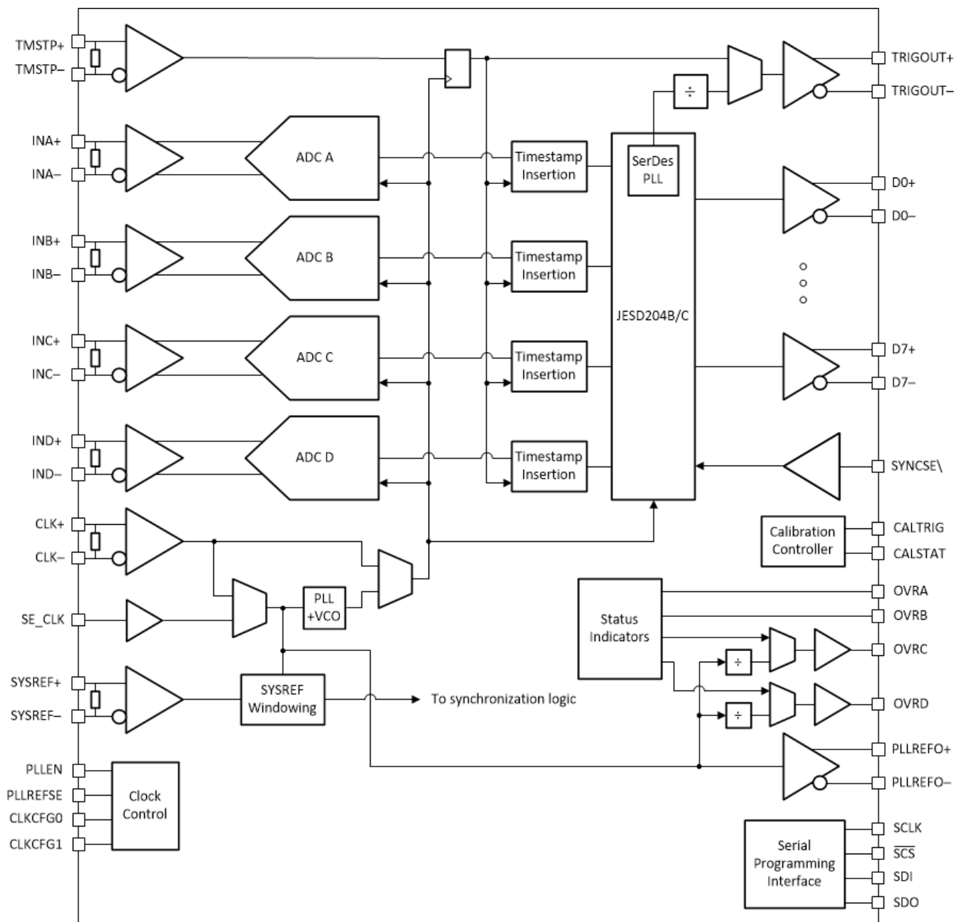
四通道器件方框图
