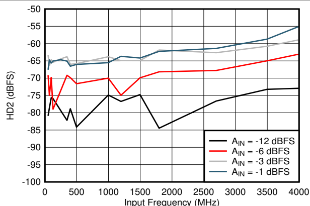
图 5-19. HD2 vs Input Frequency
