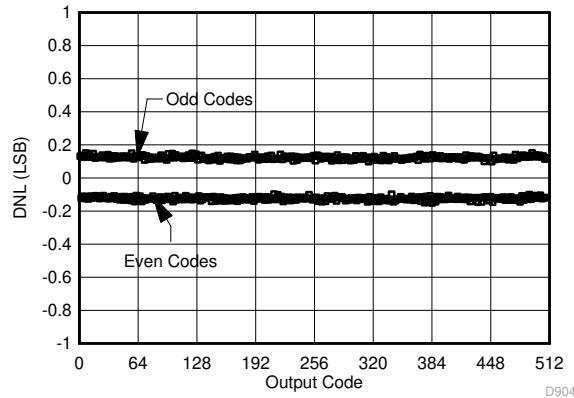
图 5-1. DNL vs Code
