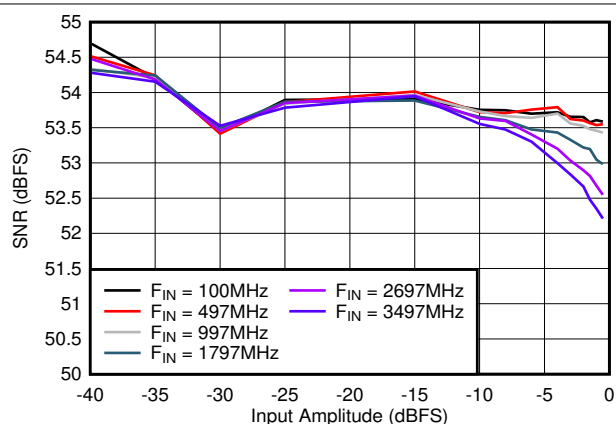
图 5-30. SNR vs Input Amplitude
