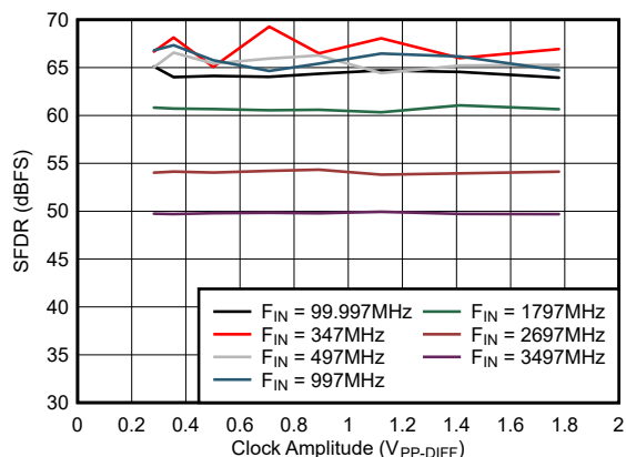
图 5-33. SFDR vs Clock Amplitude
