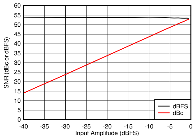
图 5-32. SNR vs Input Amplitude
