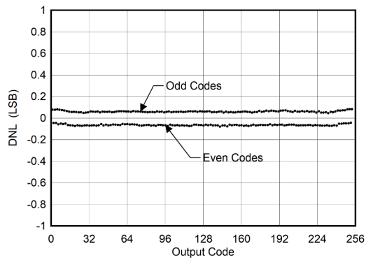
图 5-3. DNL vs ADC Code
