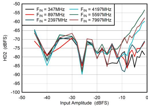
图 5-61. DES Mode: HD2 vs Input Amplitude
