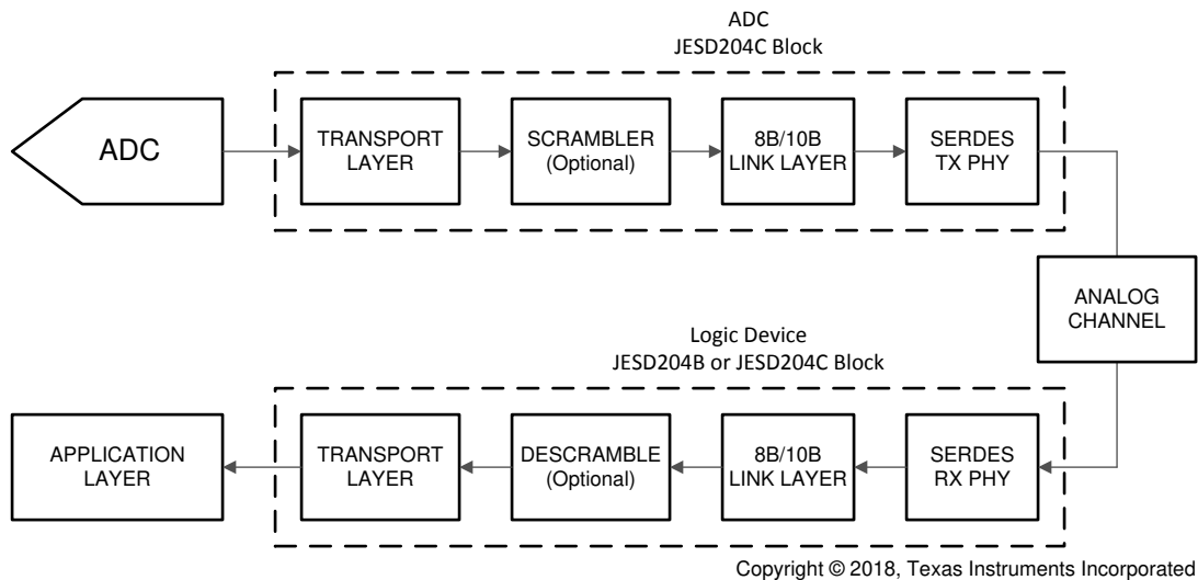
图 6-8. Simplified 8B/10B Encoded JESD204C Interface Diagram
