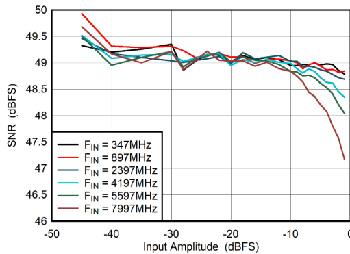
图 5-57. DES Mode: SNR vs Input Amplitude
