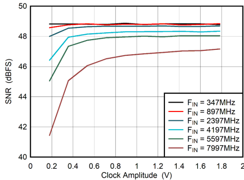
图 5-81. DES Mode: SNR vs Clock Amplitude
