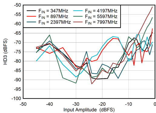
图 5-63. DES Mode: HD3 vs Input Amplitude
