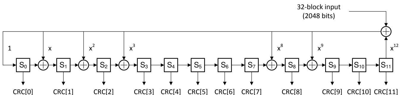
图 6-10. CRC-12 Parity Bit Generator
