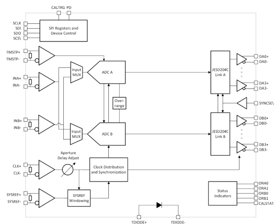
ADC08DJ5200RF 方框图
