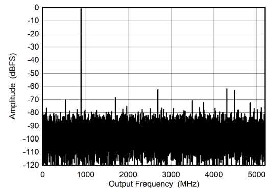
图 5-6. DES Mode: Single Tone FFT at 897 MHz
