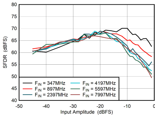
图 5-59. DES Mode: SFDR vs Input Amplitude
