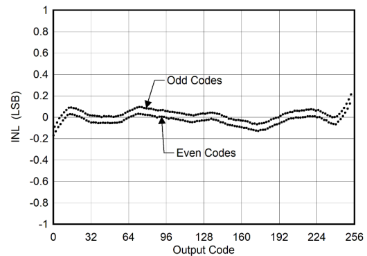
图 5-4. INL vs ADC Code
