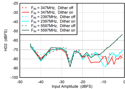
图 5-62. DES Mode: HD2 vs Input Amplitude and Dither
