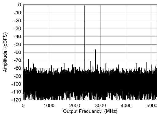
图 5-7. DES Mode: Single Tone FFT at 2397 MHz
