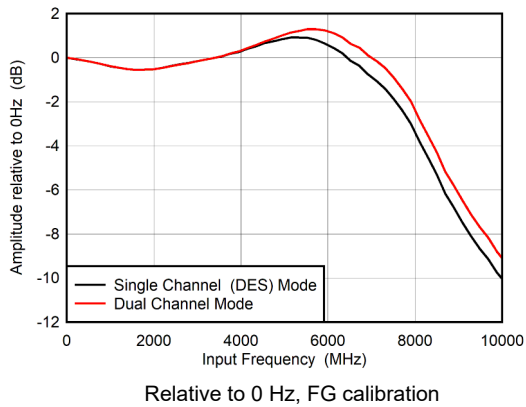
图 5-1. Input Amplitude vs Input Frequency
