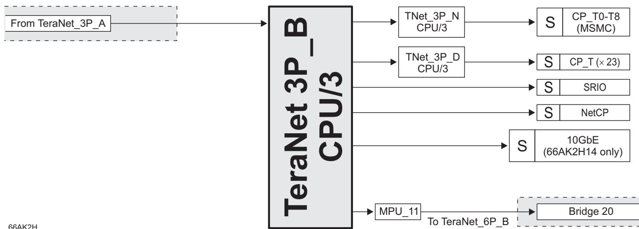
图 9-6. TeraNet 3P_B
