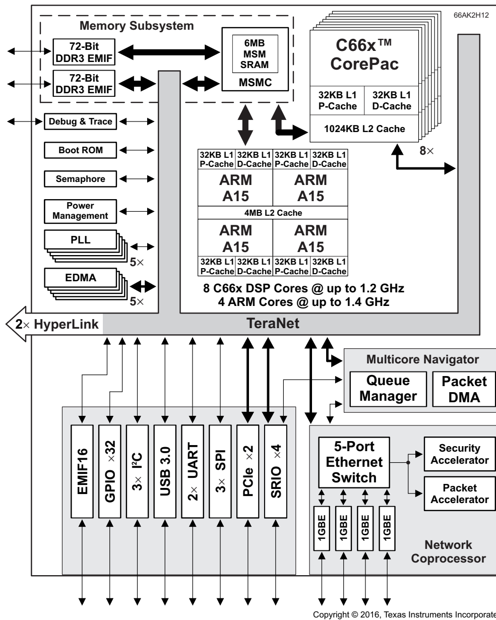
图 1-2. 功能方框图 (66AK2H12)
