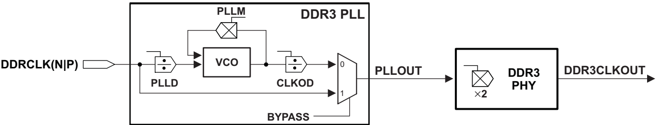
图 11-22. DDR3 PLL Block Diagram
