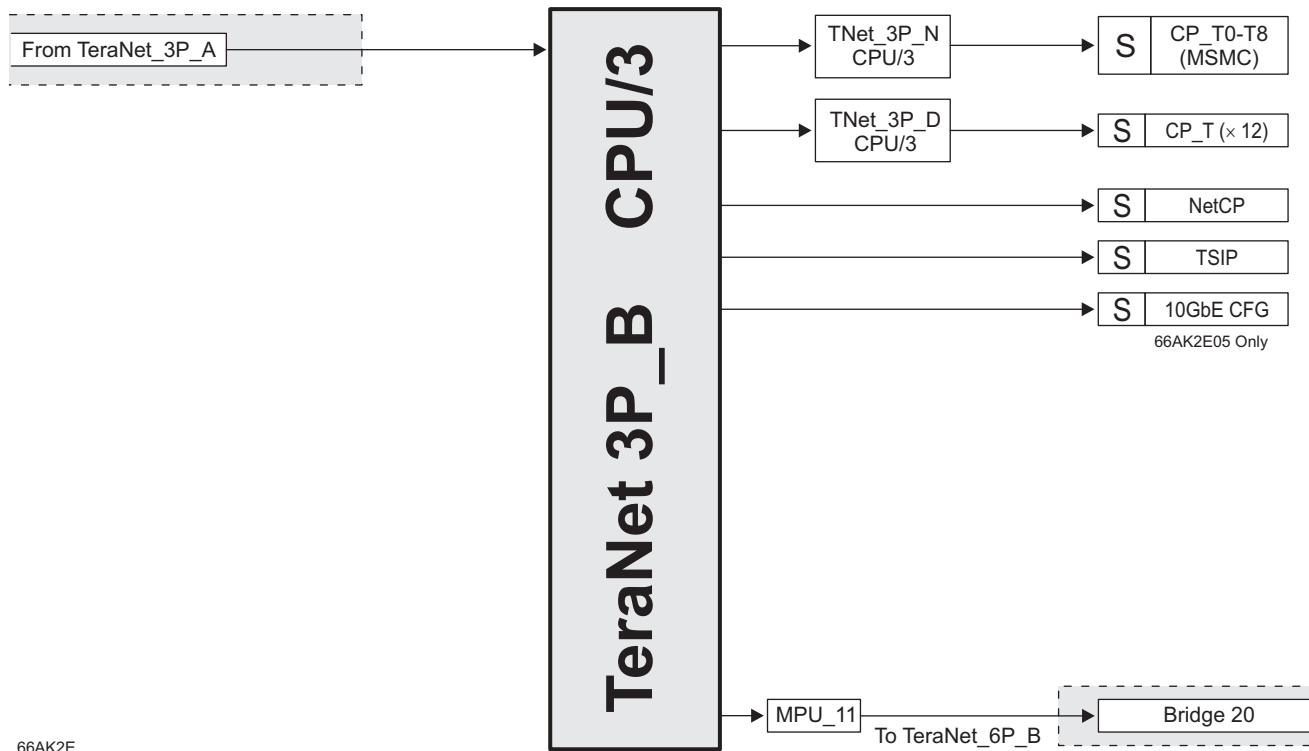
图 8-6. TeraNet 3P_B
