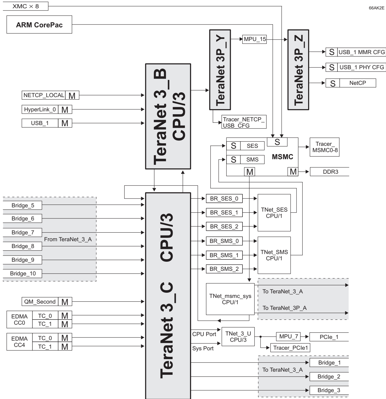
图 8-3. TeraNet 3_C
