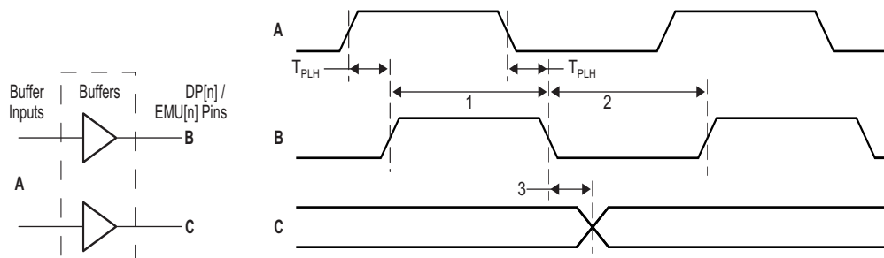
图 11-56. Trace Timing
