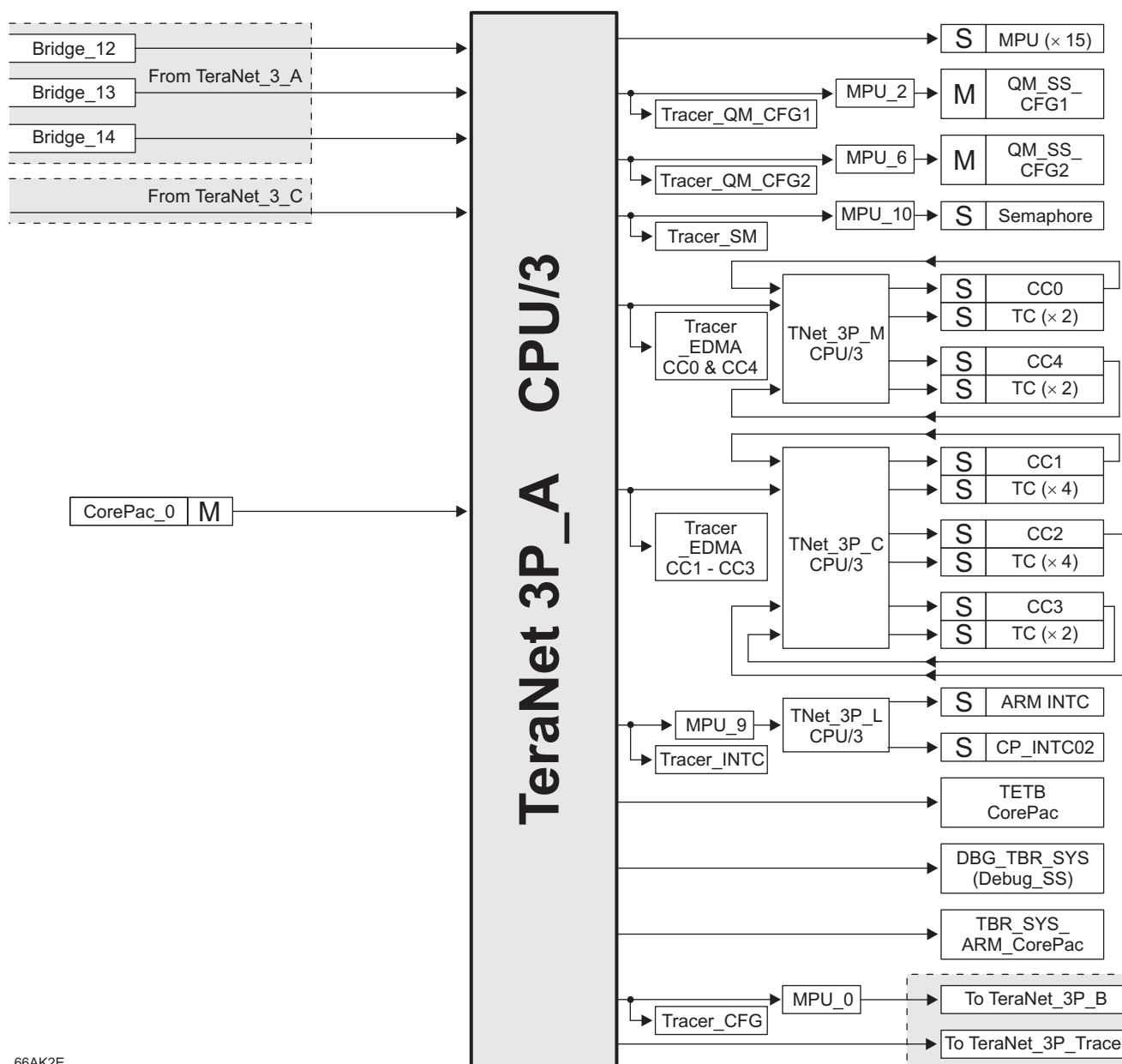
图 8-5. TeraNet 3P_A
