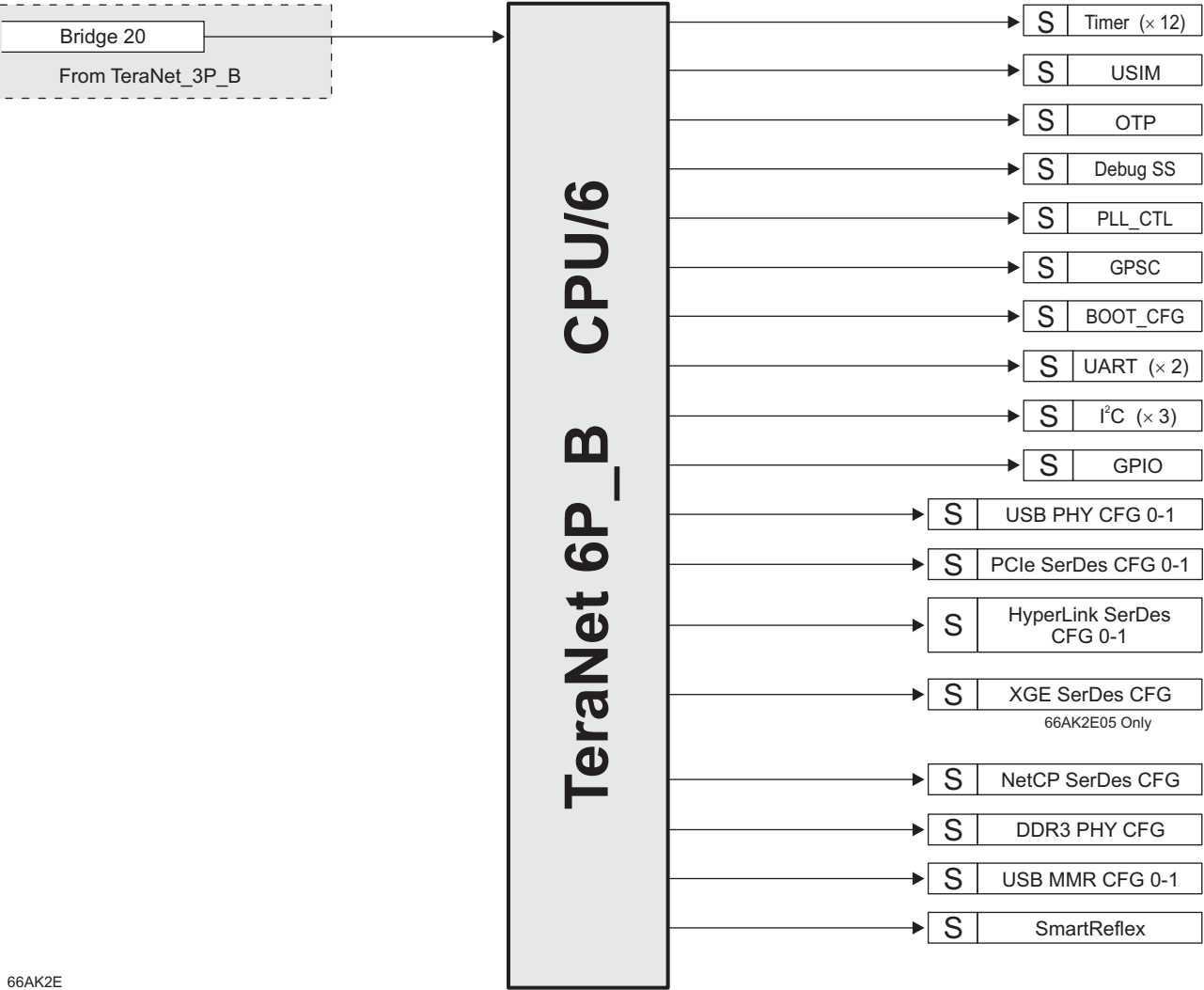
图 8-7. TeraNet 6P_B
