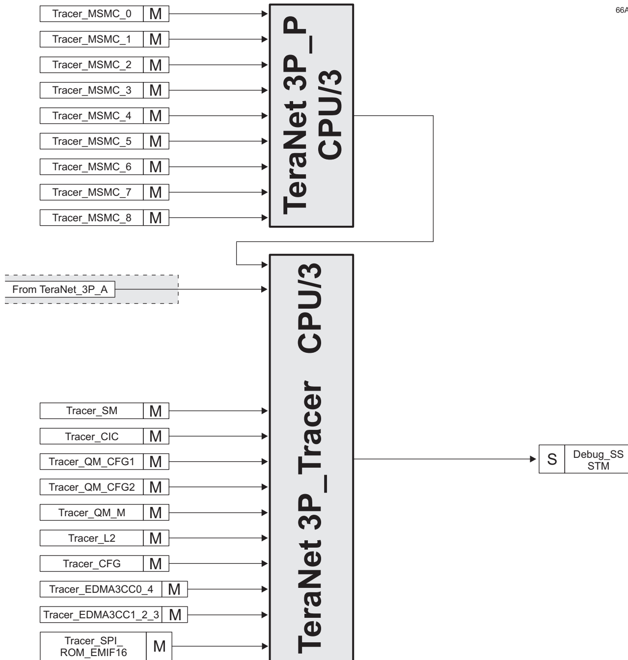
图 8-8. TeraNet 3P_Tracer
