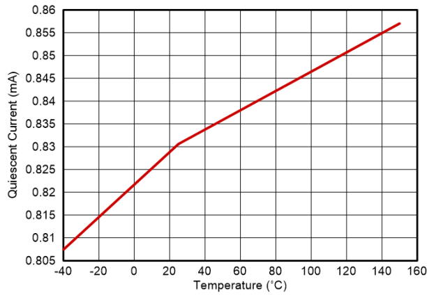
图 5-5. 静态电流
