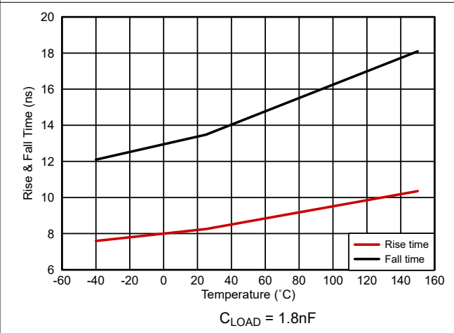
图 5-16. 输出上升和下降时间 C LOAD = 1.8nF
