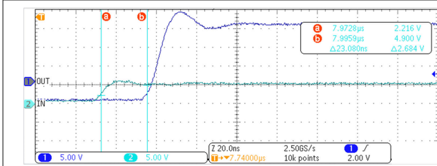
图 7-3. UCC57102Z 上升 (导通) 传播延迟
