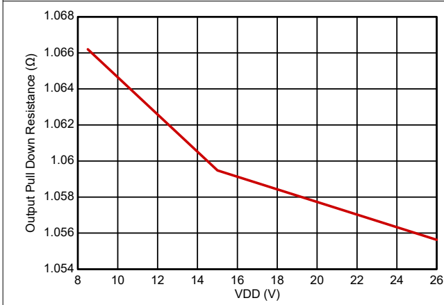
图 5-13. 输出下拉电阻
