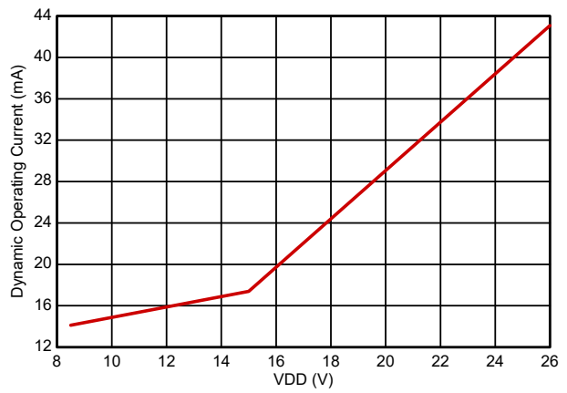
图 5-8. 工作电源电流
