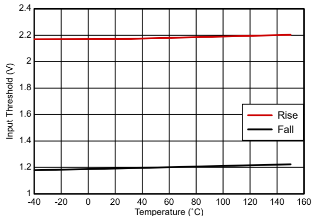
图 5-10. 输入阈值
