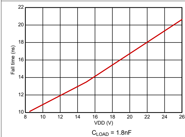
图 5-15. 输出下降时间 C LOAD = 1.8nF
