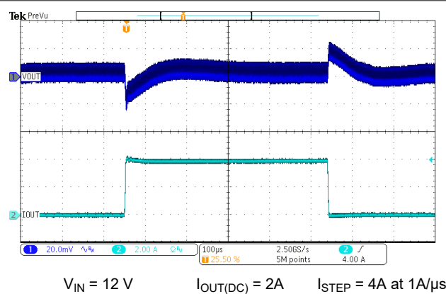
图 7-8. Load Transient
