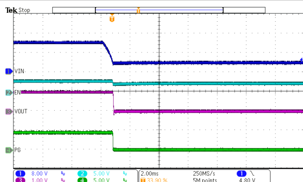
I_{OUT} = 8A 图 7-14. VIN Shutdown
