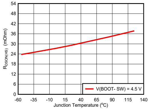
图 5-1. High-Side FET Rdson
