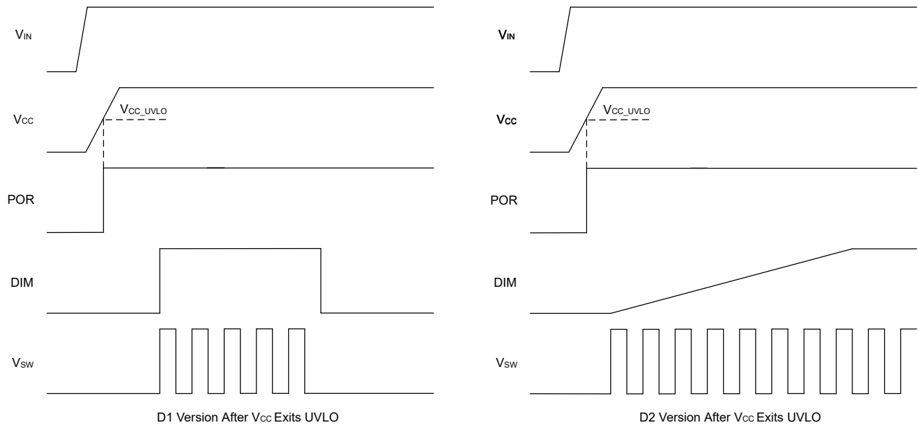
图 7-2. 启动顺序
