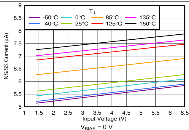
图 32. NR/SS Current vs Input Voltage
