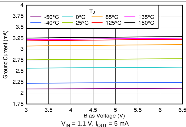
图 29. Quiescent Current vs Bias Voltage
