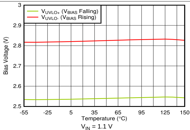
图 34. V_{BIAS} UVLO vs Temperature
