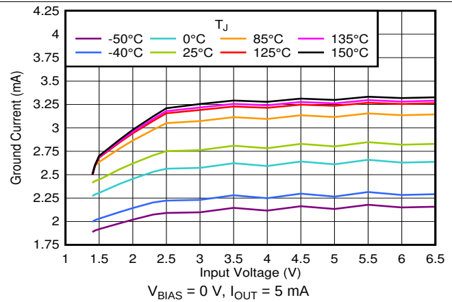
图 28. Quiescent Current vs Input Voltage
