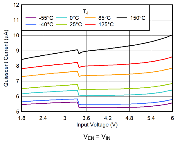
图 6-8. I_Q vs V_{IN}
