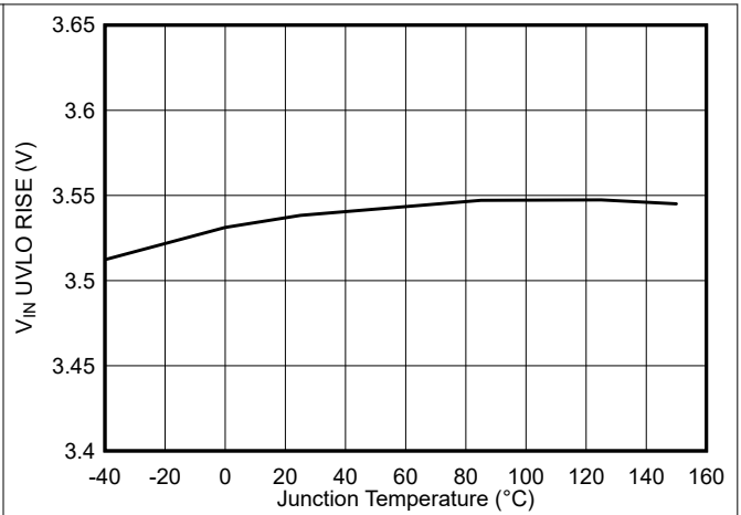
图 8-8. V IN UVLO 上升阈值与结温间的关系
