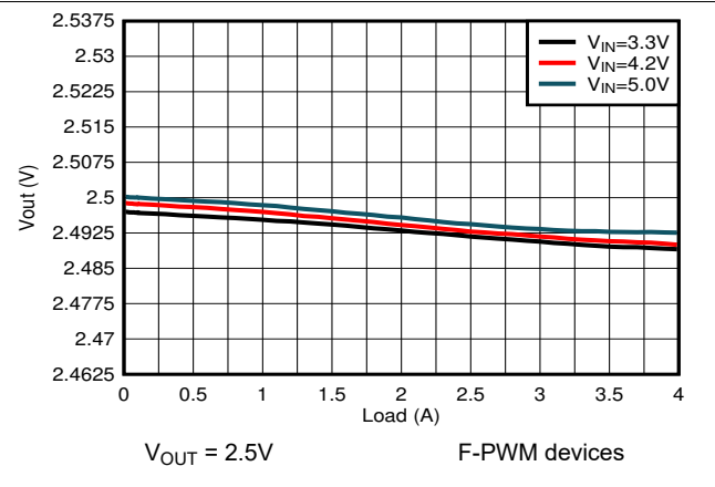
图 8-18. Load Regulation
