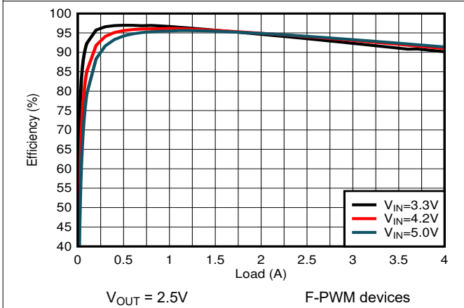
图 8-17. PWM Efficiency
