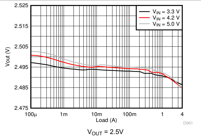
图 8-16. Load Regulation
