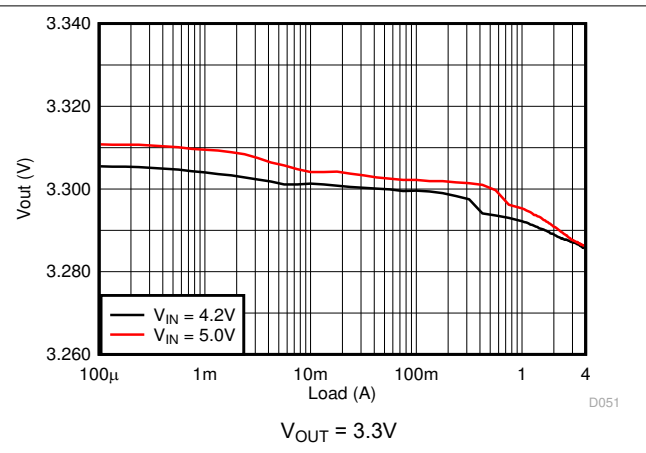
图 8-20. Load Regulation
