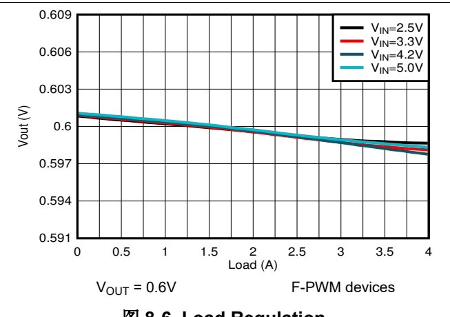
图 8-6. Load Regulation
