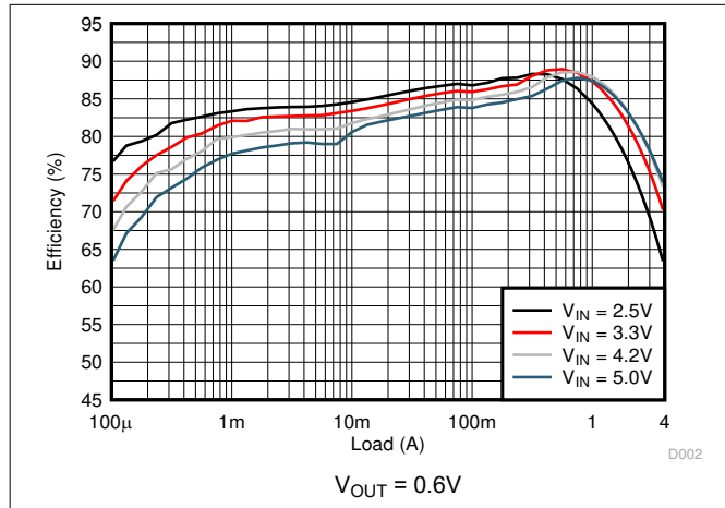
图 8-3. Efficiency
