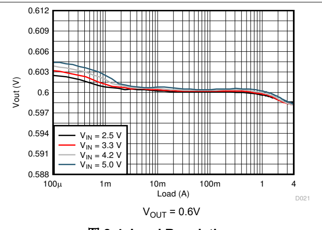
图 8-4. Load Regulation
