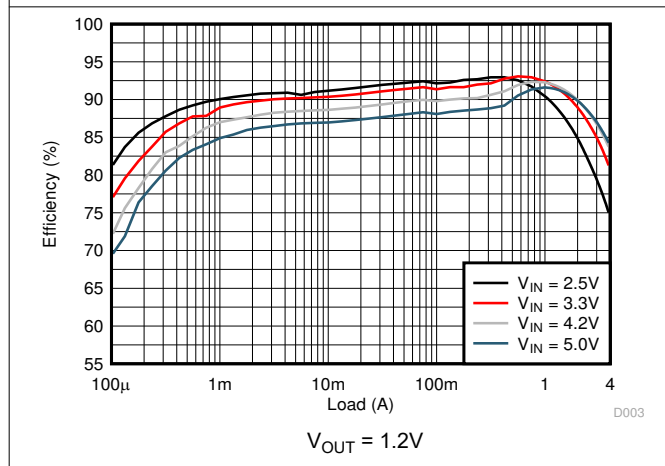
图 8-7. Efficiency
