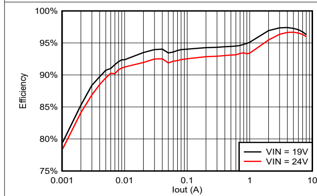
图 5-21. TPS56837 效率, V_{out} = 12V , F_{sw} = 800kHz
