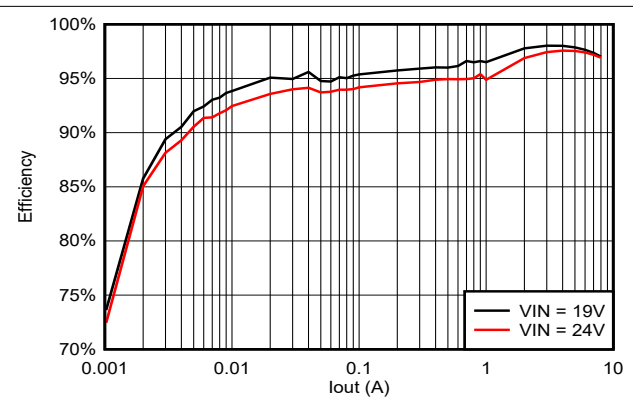
图 5-20. TPS56837 效率, V_{out} = 12V , F_{sw} = 500kHz
