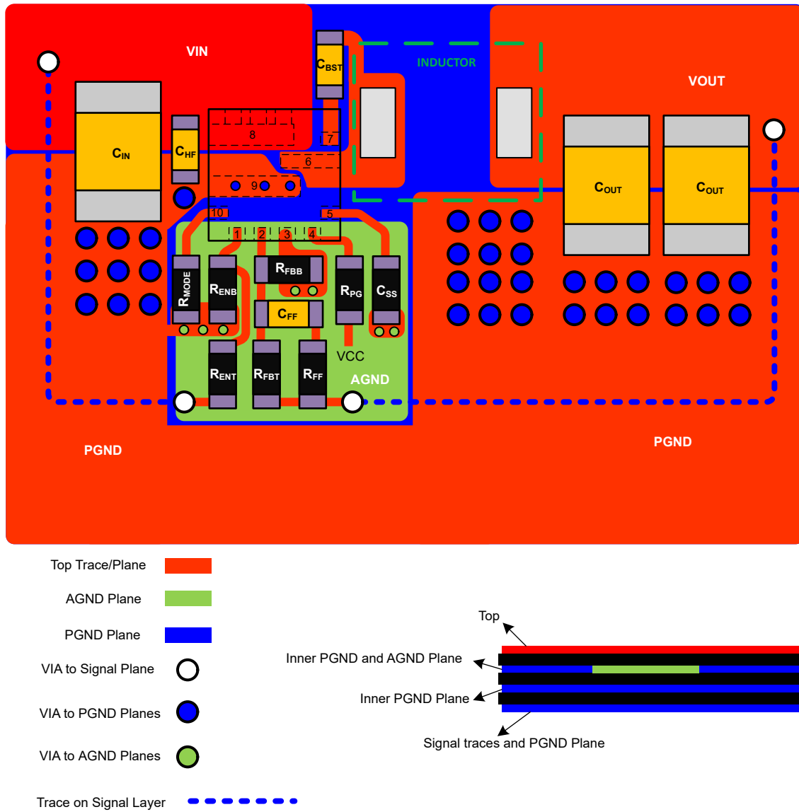
图 7-18. TPS56837 布局
