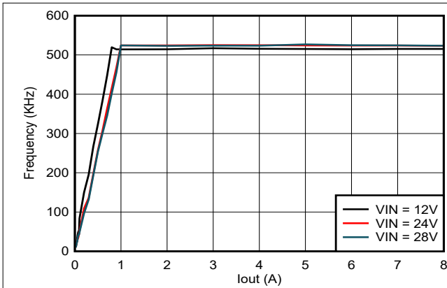
图 5-13. TPS56837 开关频率与输出电流间的关系, V_{out} = 5V , F_{sw} = 500kHz
