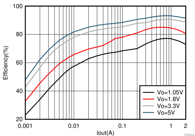
TPS562231 效率
