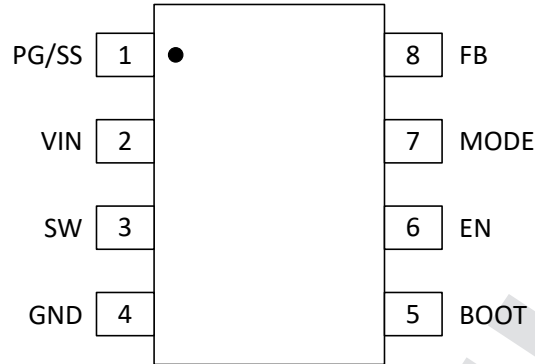
图 5-1. 8 引脚 SOT583 DRL 封装 (俯视图)
