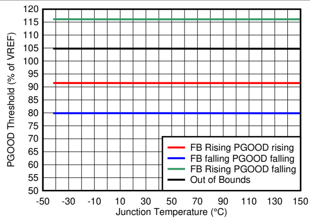
图 5-9. PGOOD 阈值
