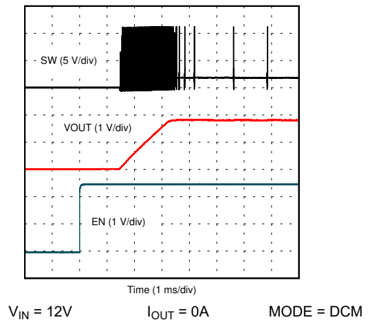
图 7-17. EN 启动 - DCM
