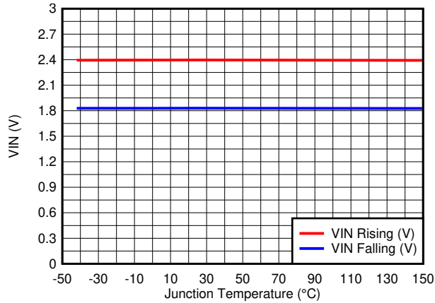
图 5-7. VIN UVLO
