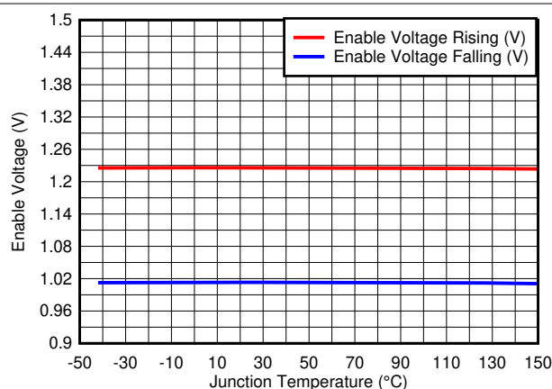
图 5-5. 使能电压
