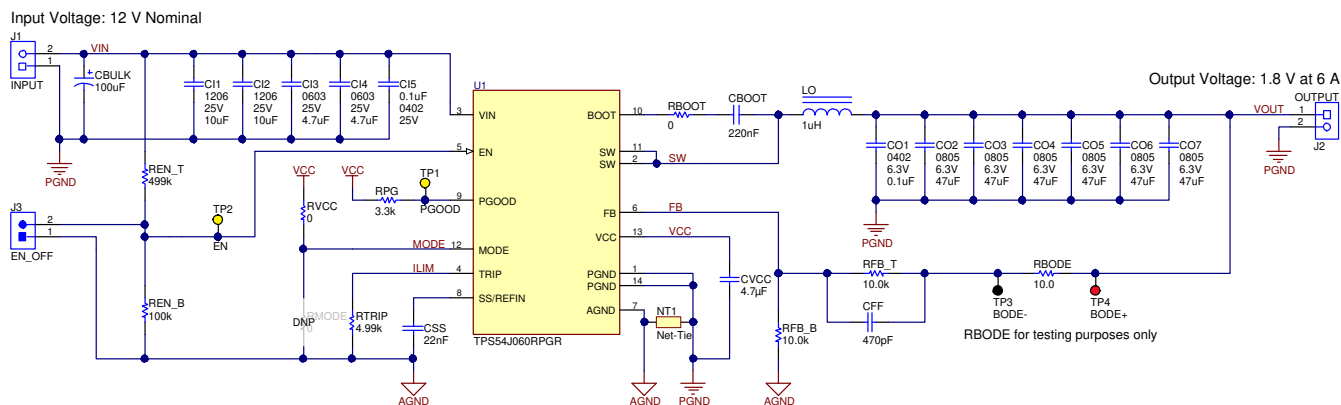
图 7-1. 应用电路图
