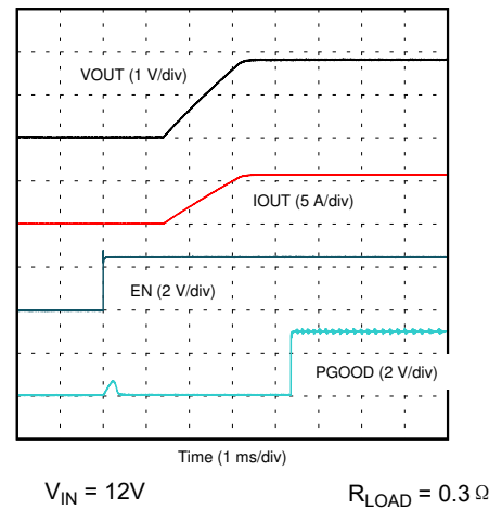
图 7-15. EN 启动
