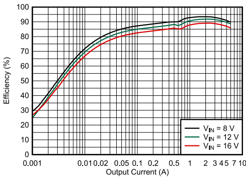
图 7-4. 效率 - 1100kHz , FCCM , 外部 3.3V VCC , 4.7\ \Omega R_{BOOT}
