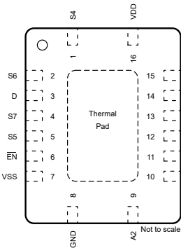
图 6-3. TMUX4051-Q1 BQB 封装，16 引脚 WQFN (顶视图)
