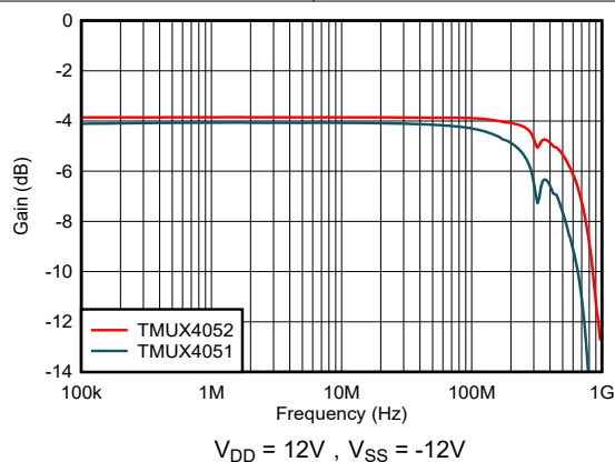
图 7-9. 导通响应与频率之间的关系
