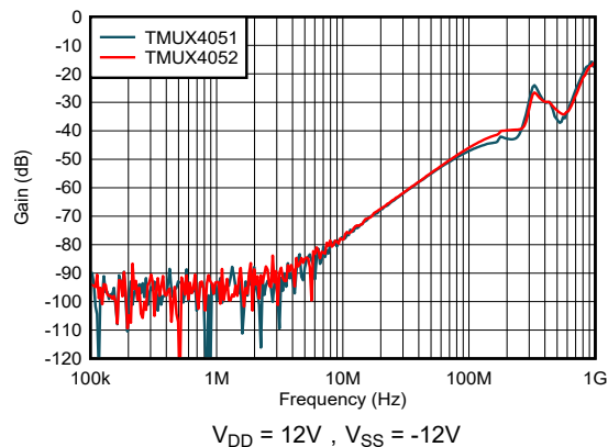
图 7-8. 关断隔离与频率之间的关系
