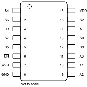
图 6-2. TMUX4051-Q1 DYY 封装，16 引脚 SOT-23-THIN (顶视图)
