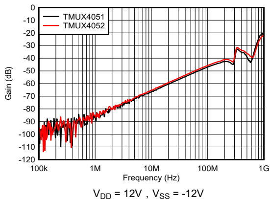
图 7-7. Xtalk 与频率之间的关系
