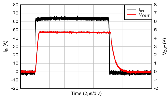
图 6-13. 电流过载响应
