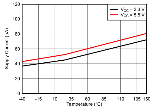
图 5-8. Low Power Mode Current
