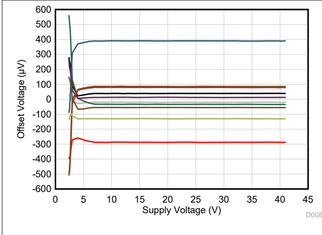
图 5-9. 失调电压与电源间的关系
