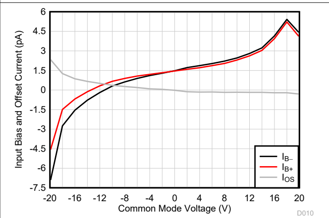
图 5-12. 输入偏置电流与共模电压间的关系
